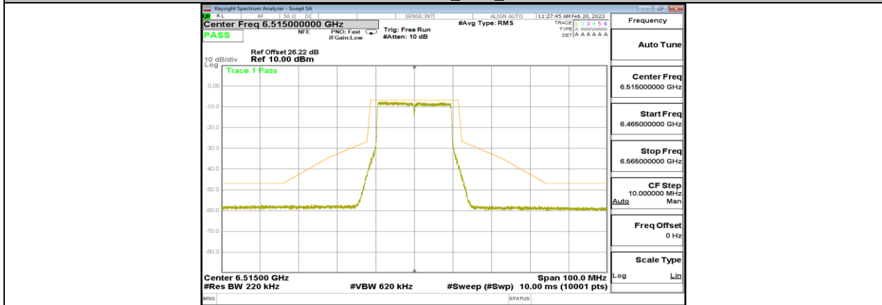
11BE20MIMO_Ant2_6515
