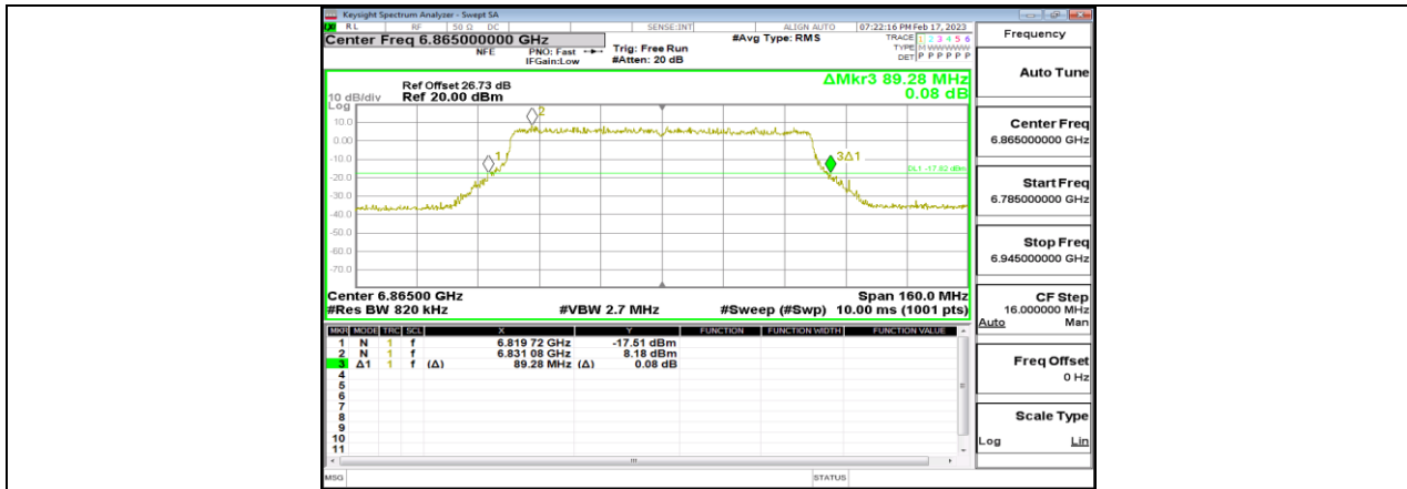
11BE80MIMO_Ant4_6865
