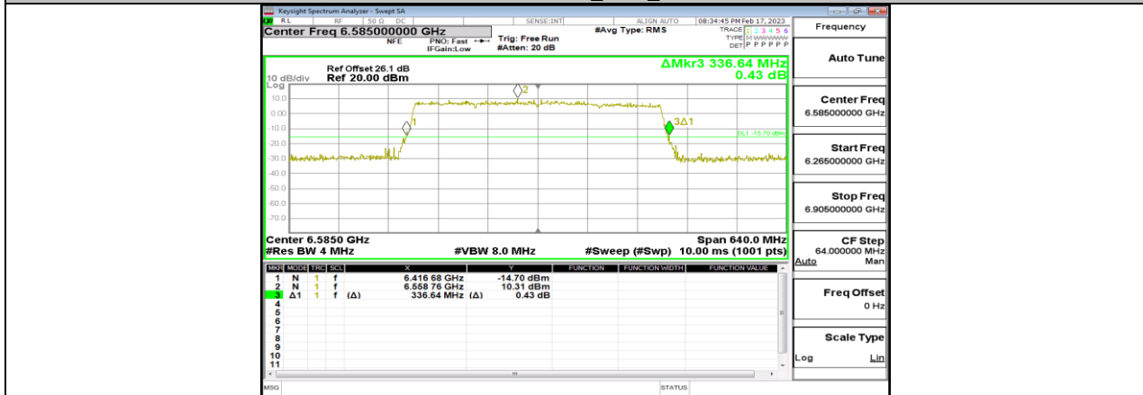
11BE320MIMO_Ant2_6585
