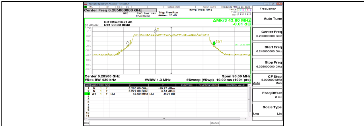
11BE40MIMO_Ant2_6285
