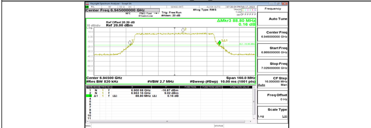
11BE80MIMO_Ant4_6945
