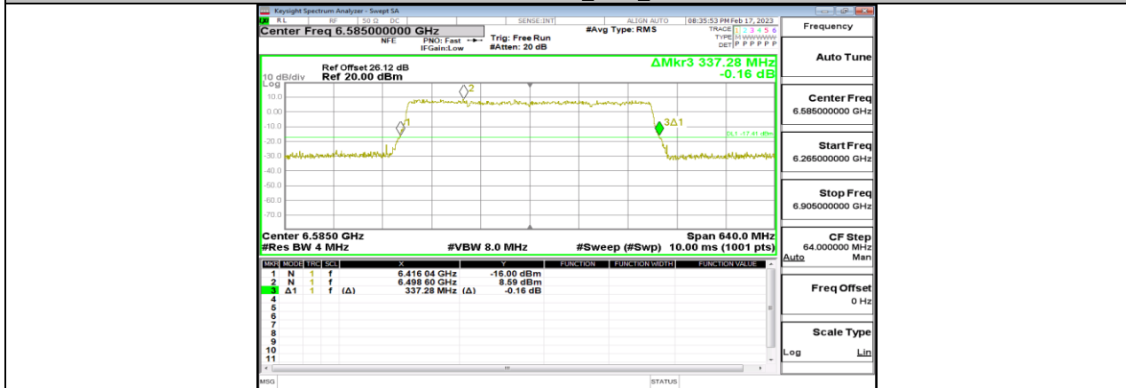
11BE320MIMO_Ant4_6585
