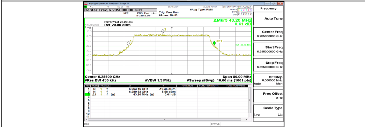
11BE40MIMO_Ant4_6285
