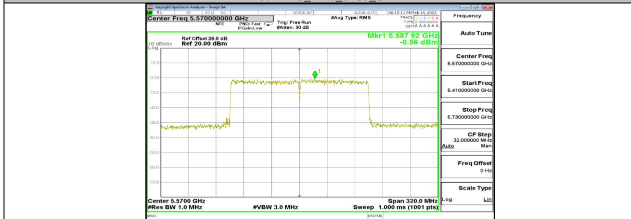
11BE160MIMO_Ant1_5570
