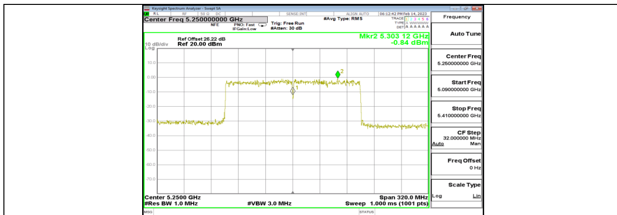
11BE160MIMO_Ant3_5250_UNII-2A
