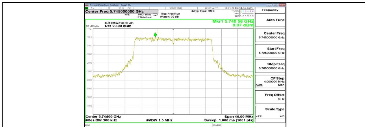
11BE20MIMO_Ant1_5745
