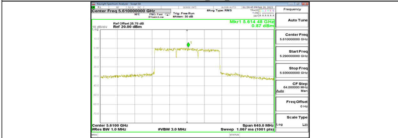
11BE240MIMO_Ant3_5610
