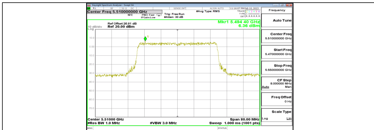
11BE40MIMO_Ant3_5510
