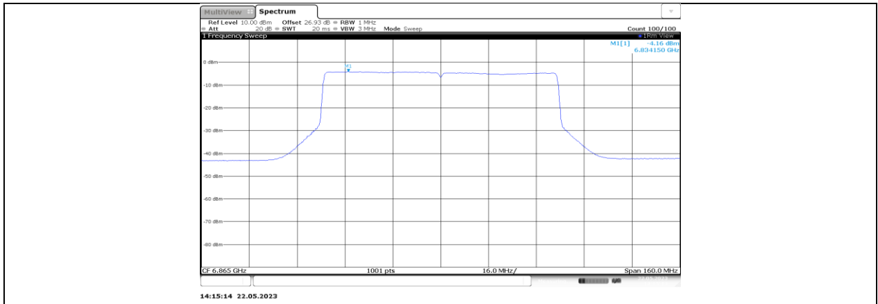
11BE80MIMO_Ant6_6865
