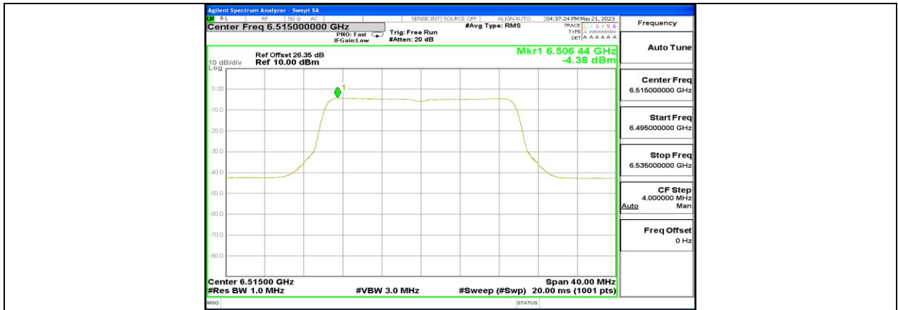
11BE20MIMO_Ant6_6515
