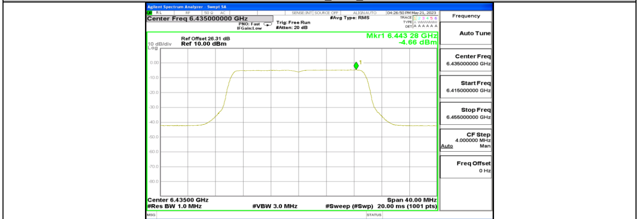
11BE20MIMO_Ant3_6435
