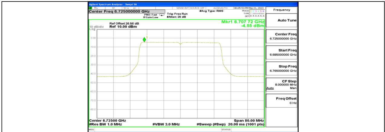
11BE40MIMO_Ant6_6725
