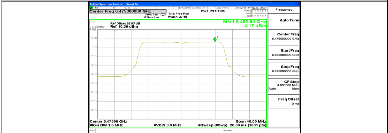
11BE20MIMO_Ant6_6475
