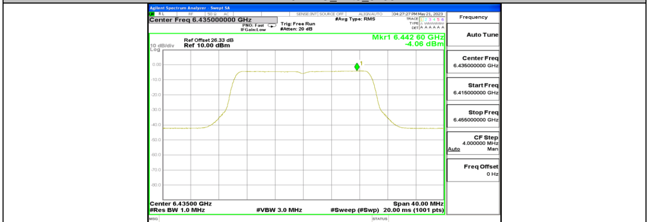
11BE20MIMO_Ant6_6435
