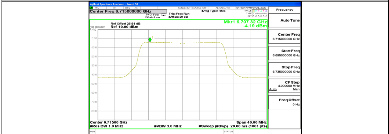
11BE20MIMO_Ant6_6715
