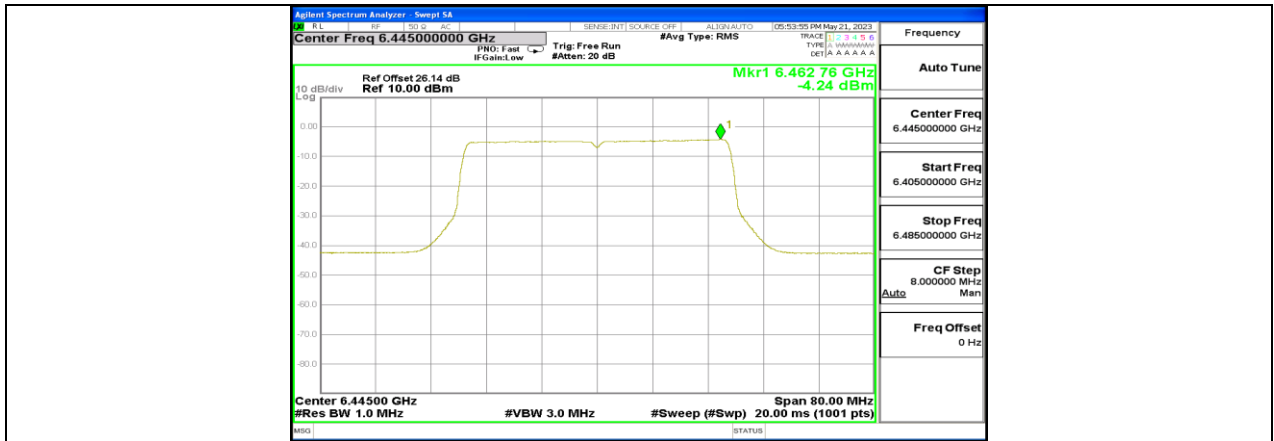
11BE40MIMO_Ant6_6445
