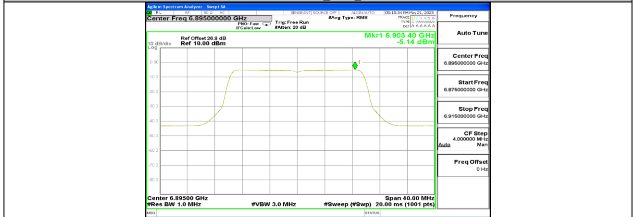
11BE20MIMO_Ant3_6895
