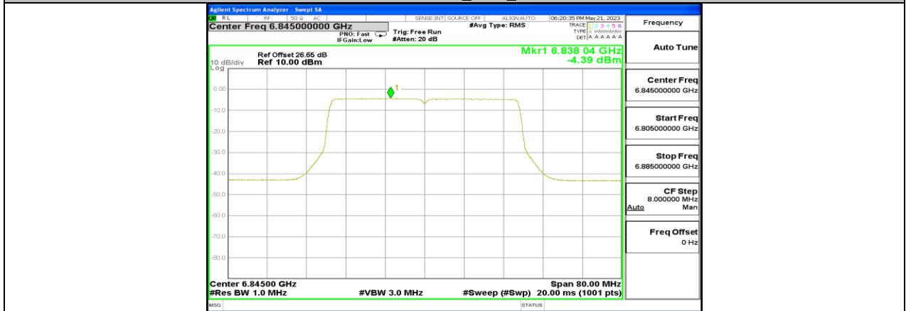
11BE40MIMO_Ant6_6845
