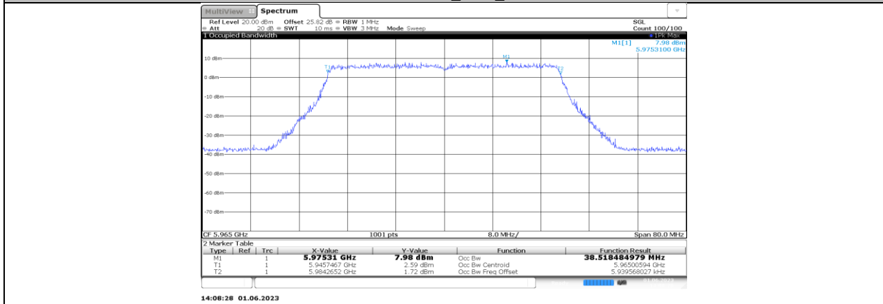
11AX40MIMO_Ant6_5965
