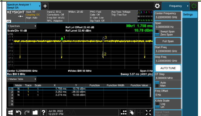
802.11ax-HE80
