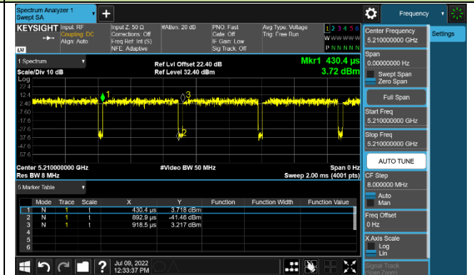
802.11ax-HE20
