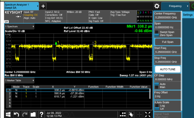
802.11ax-HE40
