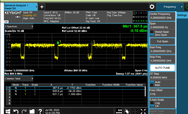
802.11ax-HE160
