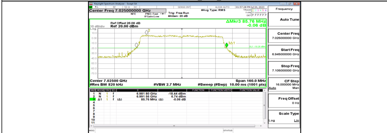
11BE80MIMO_Ant9_7025
