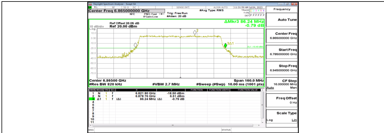
11BE80MIMO_Ant10_6865
