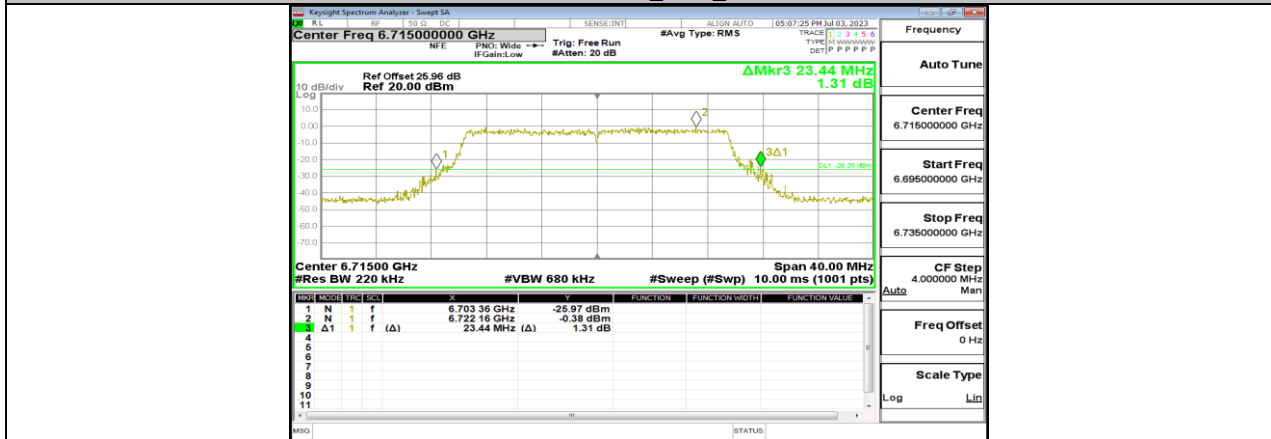
11BE20MIMO_Ant10_6715
