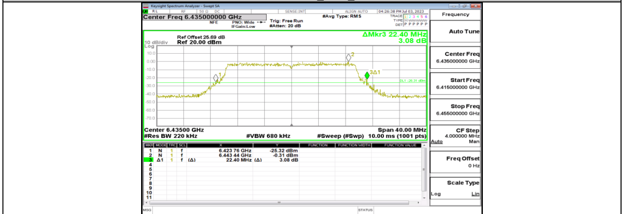
11BE20MIMO_Ant4_6435
