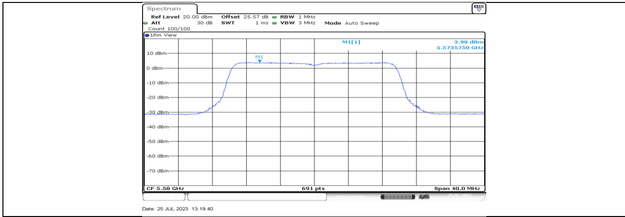
11BE20MIMO_Ant4_5580
