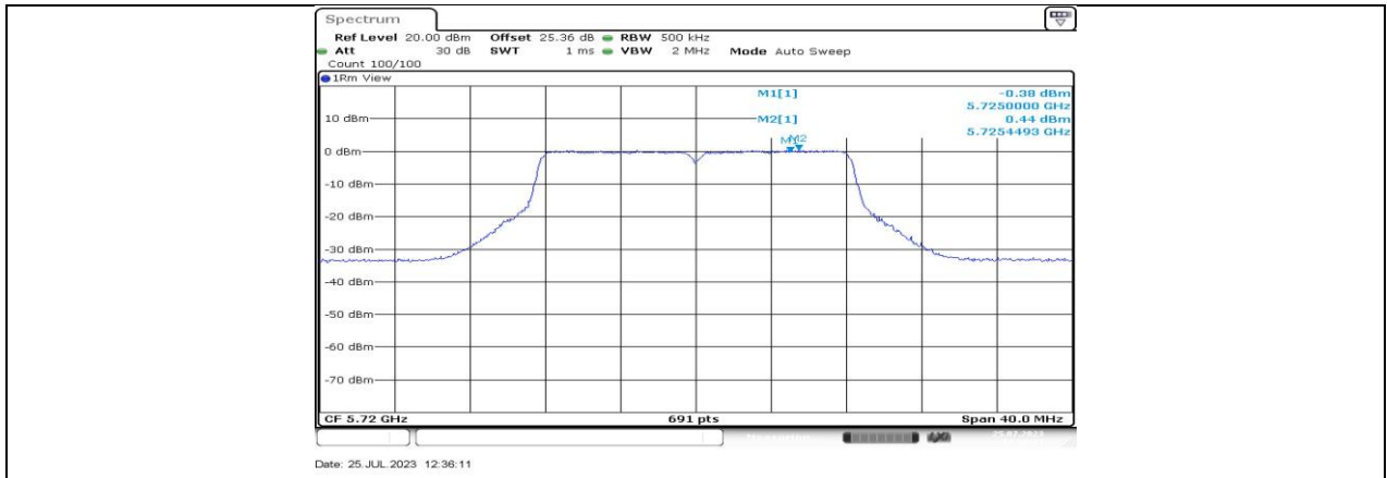
11A-CDD_Ant3_5720_UNII-3
