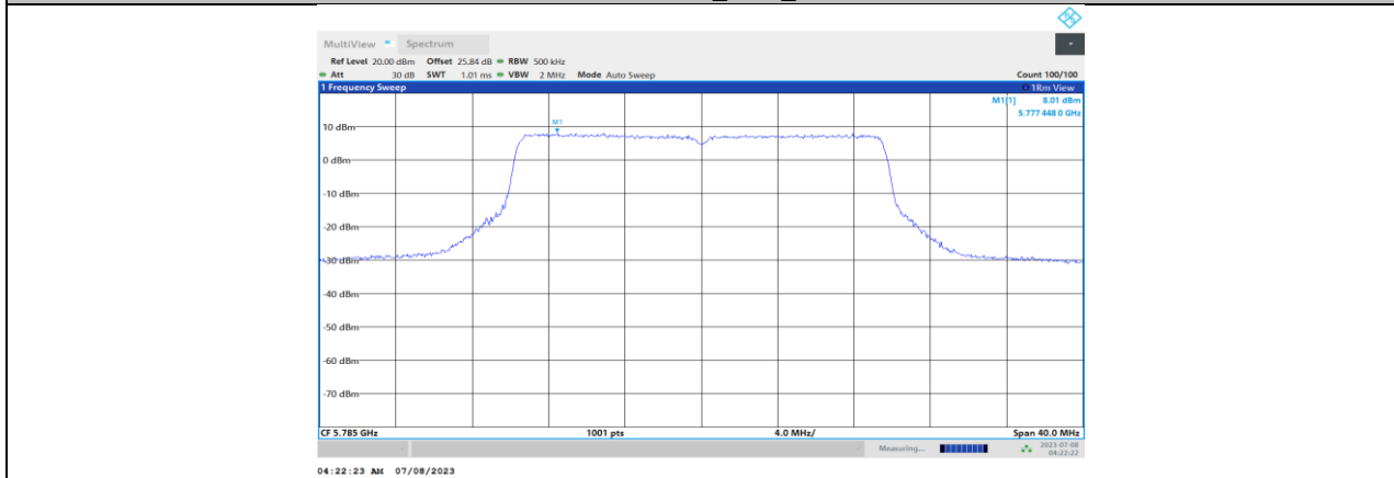
11BE20MIMO_Ant4_5785
