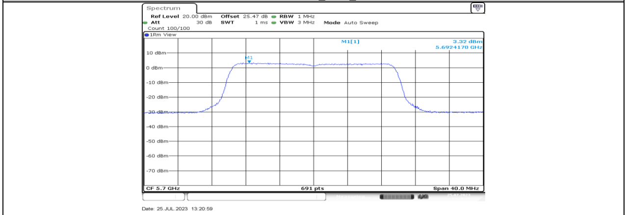
11BE20MIMO_Ant4_5700
