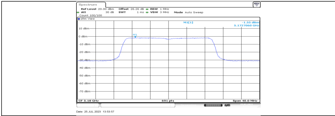
11BE20MIMO_Ant2_5180
