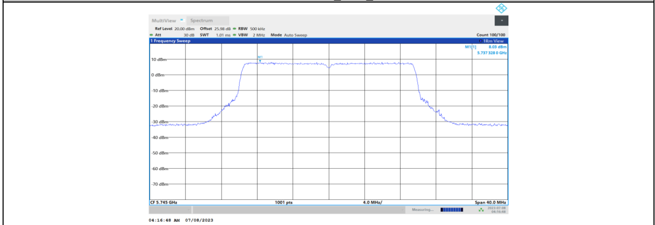
11BE20MIMO_Ant4_5745
