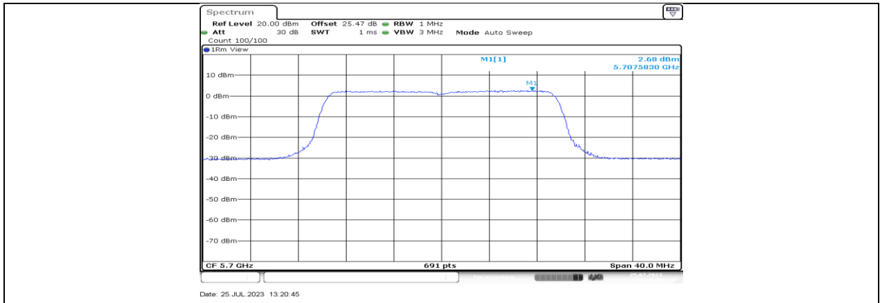
11BE20MIMO_Ant3_5700
