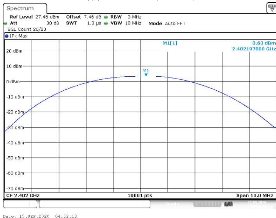
Power NVNT BLE 2402MHz Ant1
