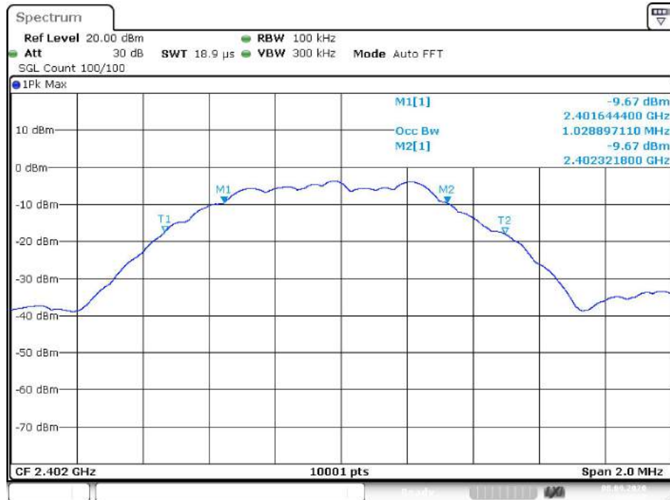
6dB NVNT BLE 2402MHz Ant1
