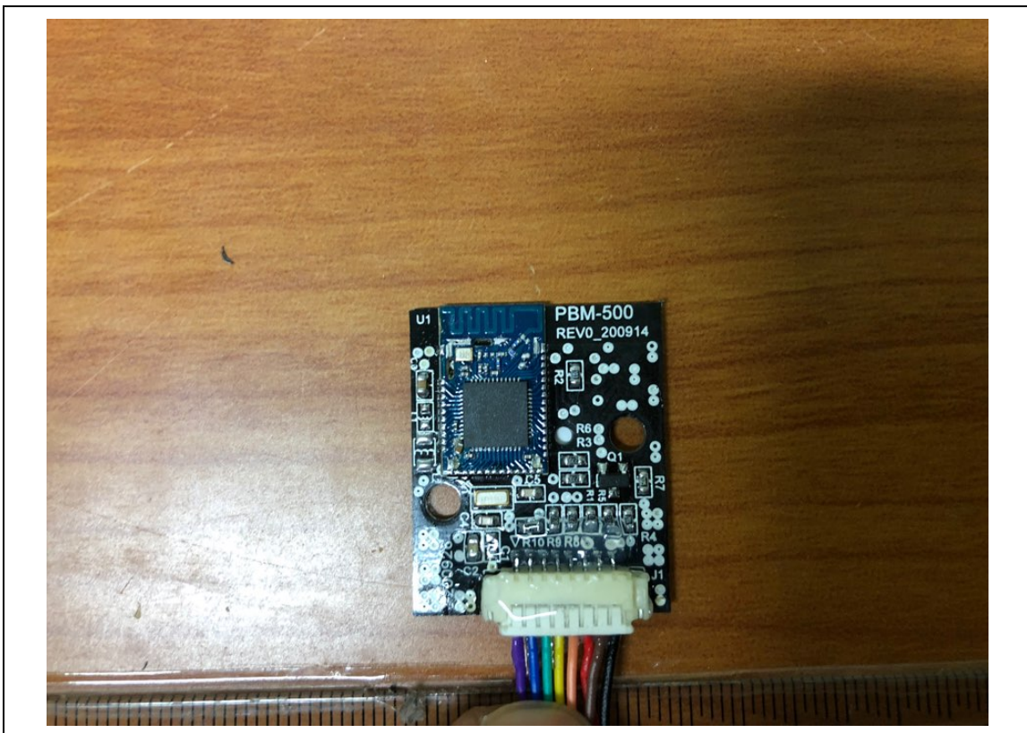
Module -Rear
