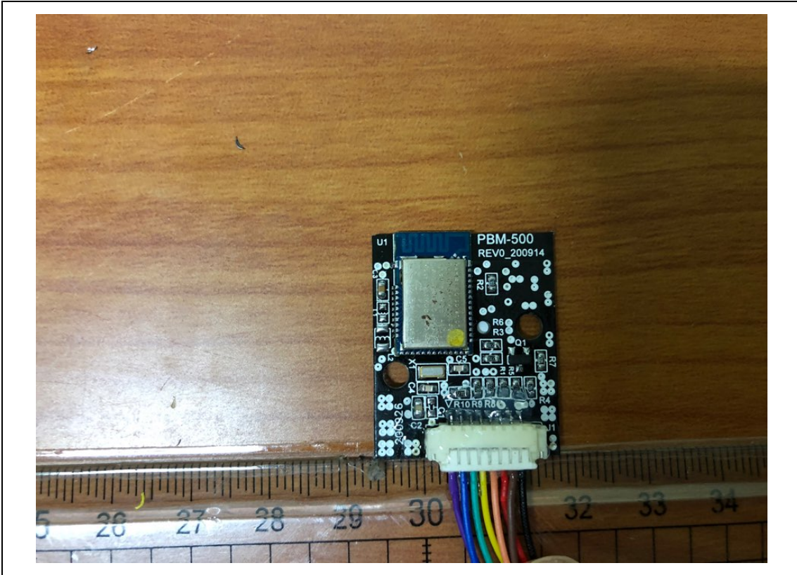
Module -Rear
