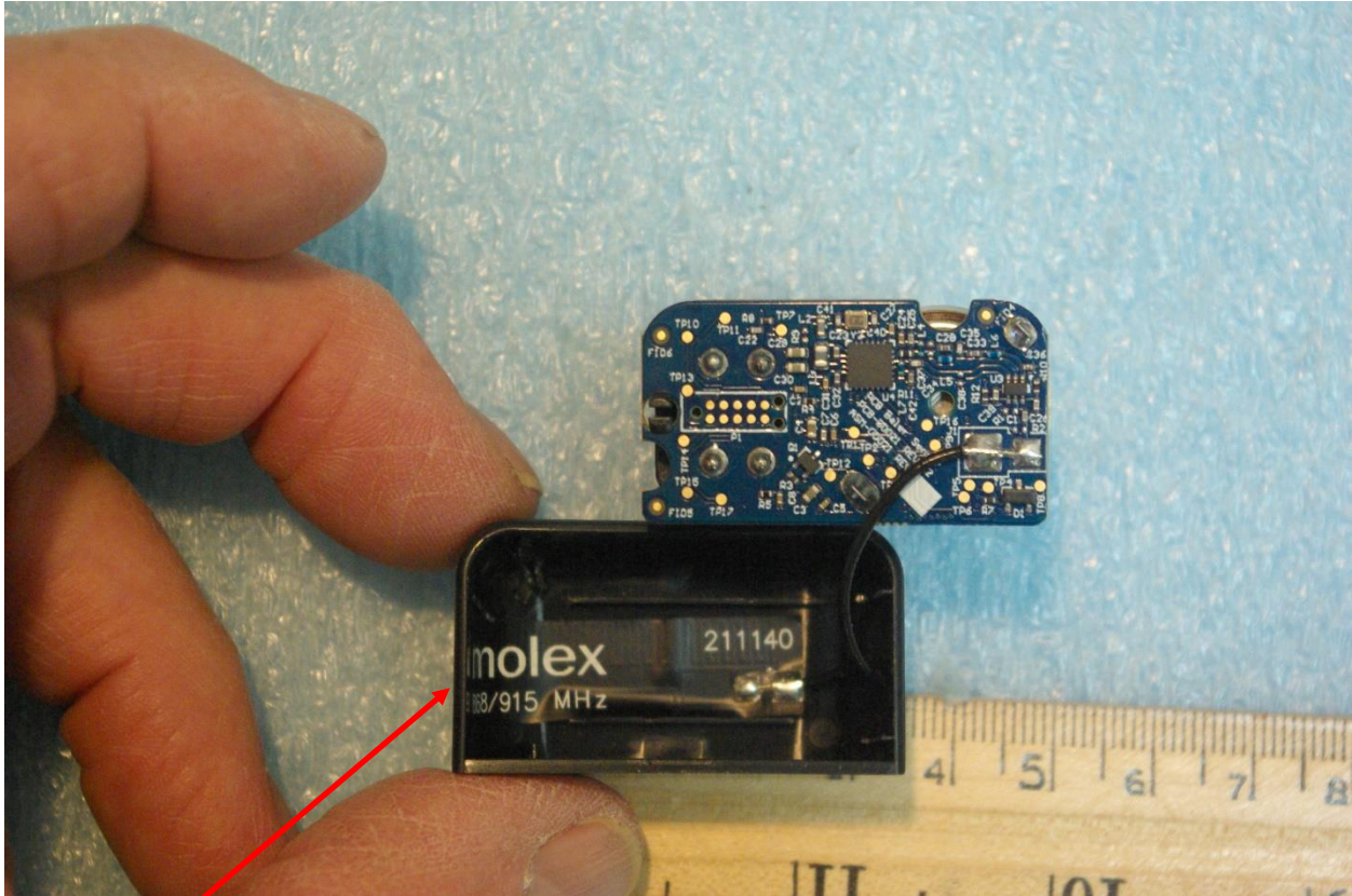
Antenna
