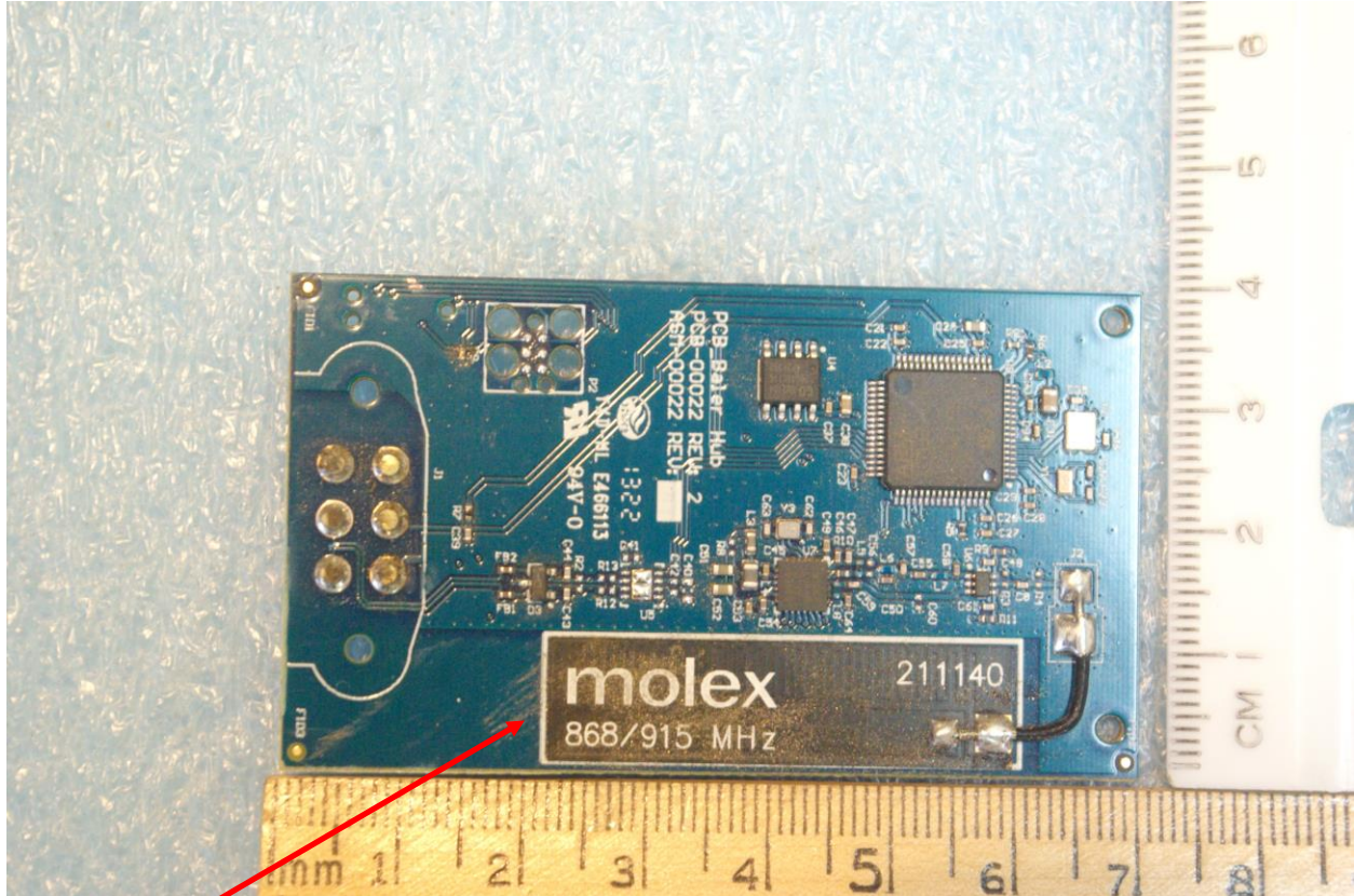
Antenna
