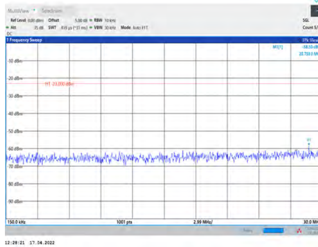
Band25-20MHz-QPSK-26140-1RB#0-Range2:0.15~30MHz
