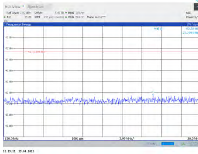
Band43-20MHz-QPSK-44690-1RB#0-Range2:0.15~30MHz
