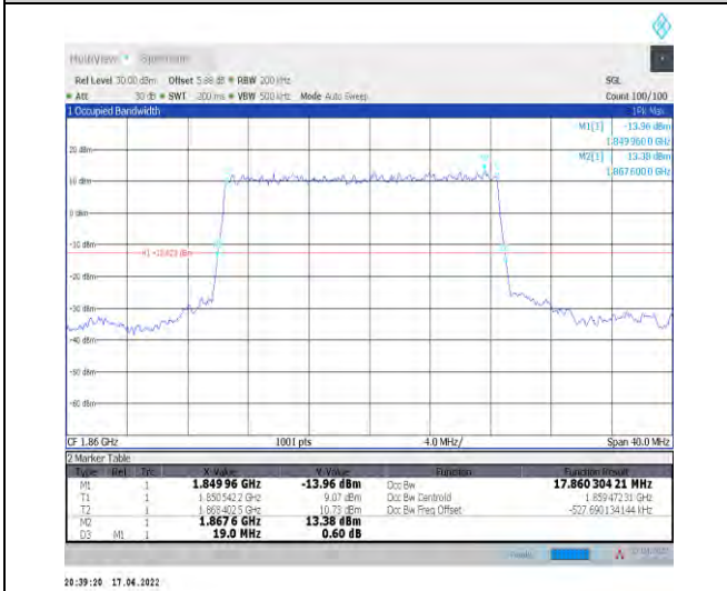
1-N2--15-20-L-2-DFT-PI2BPSK-Outer_Full-100@0-A nt1-17.86-19.000-≤20-PASS
