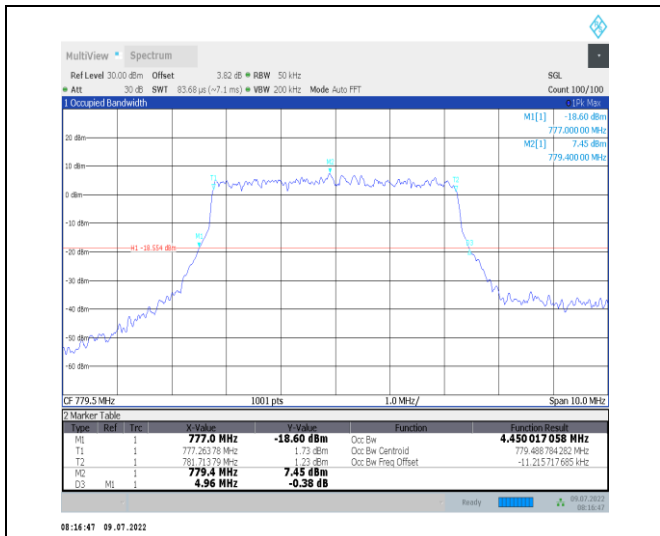
1-N13--15-5-L-9-CP-256QAM-Outer_Full-25@0-Ant1 -4.45-4.960≤5-PASS
