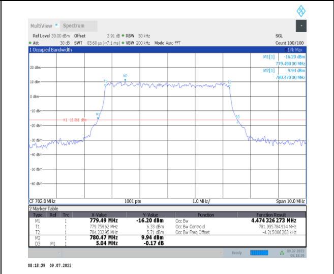
1-N13--15-5-M-7-CP-16QAM-Outer_Full-25@0-Ant1 -4.474-5.040-≤5-PASS
