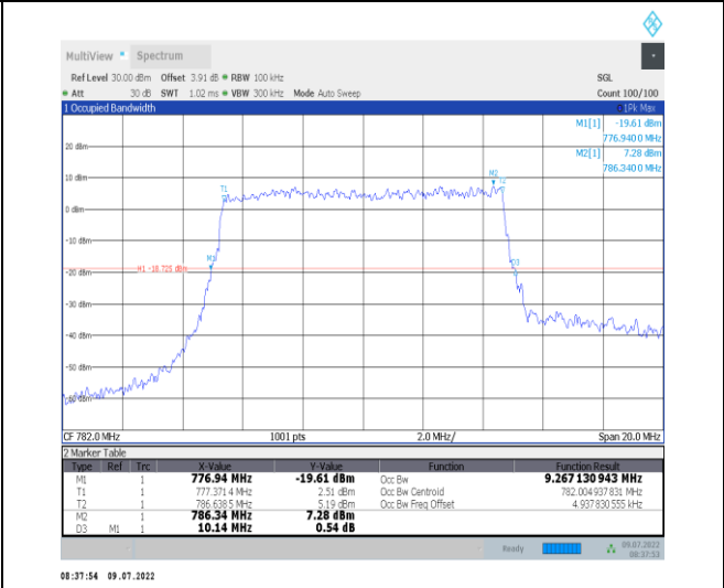
1-N13--15-10-M-9-CP-256QAM-Outer_Full-52@0-A nt1-9.267-10.140-≤10-PASS
