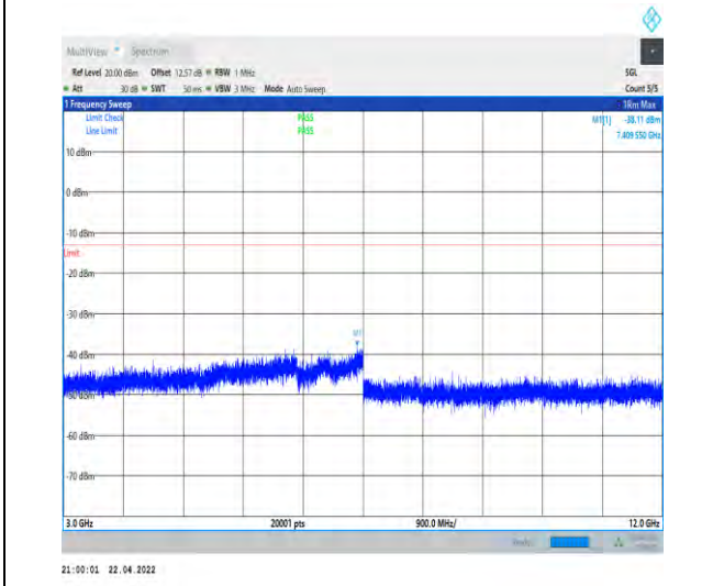
1-N66-PC3-15-40-M-1-DFT-PI2BPSK-Inner_1RB_L eft-1@1-3000-12000-Ant1--38.11--13-PASS
