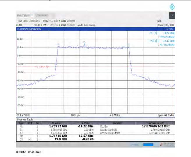
1-N66-PC3-15-20-H-3-DFT-16QAM-Outer_Full-100 @0-Ant1-17.871-19.000-≤20-PASS
