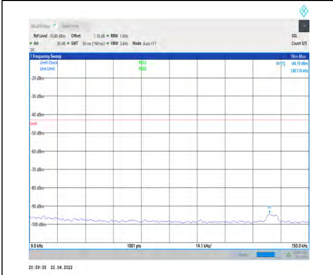
1-N66-PC3-15-40-M-1-DFT-PI2BPSK-Inner_1RB_L eft-1@1-0.009-0.15-Ant1--94.19--43-PASS
