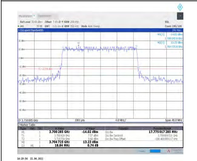
1-N77-3700-3980--30-20-L-1-DFT-QPSK-Outer_Full -50@0-Ant1-17.775-18.840-≤20-PASS
