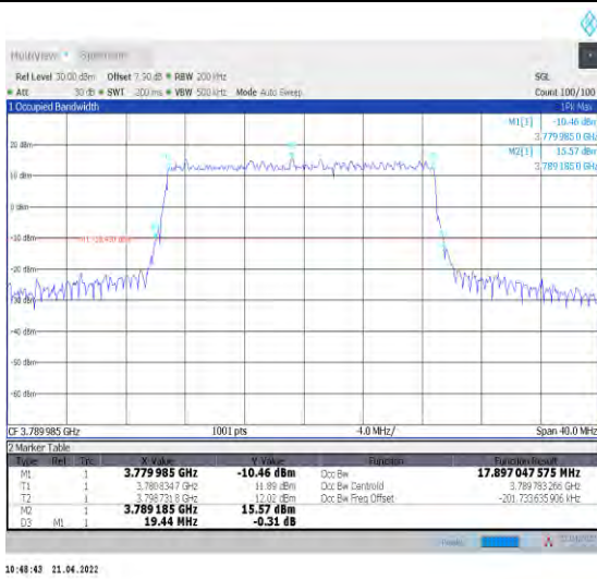
1-N78-3700-3800--30-20-H-1-DFT-QPSK-Outer_Full -50@0-Ant1-17.897-19.440-≤20-PASS
