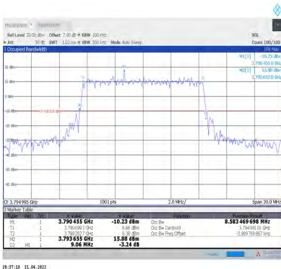
1-N78-3700-3800--30-10-H-1-DFT-QPSK-Outer_Full -24@0-Ant1-8.583-9.060-≤10-PASS
