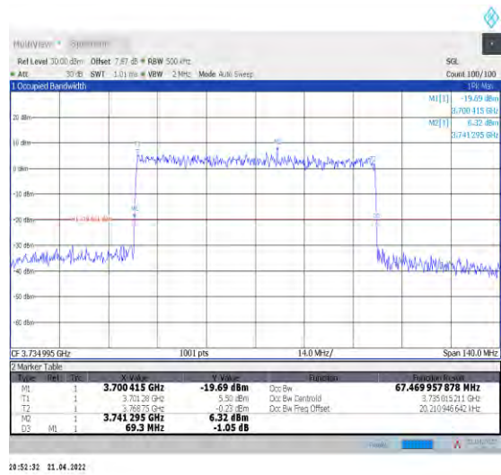
1-N78-3700-3800--30-70-L-9-CP-256QAM-Outer_Fu II-189@0-Ant1-67.47-69.300-≤70-PASS
