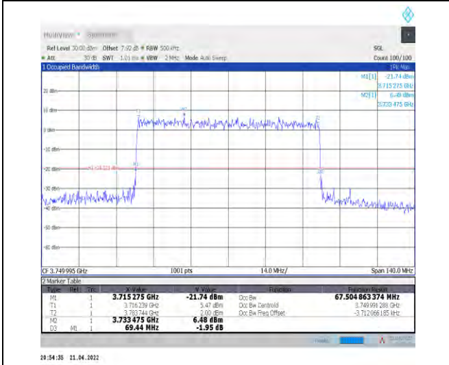
1-N78-3700-3800--30-70-M-9-CP-256QAM-Outer_F ull-189@0-Ant1-67.505-69.440-≤70-PASS
