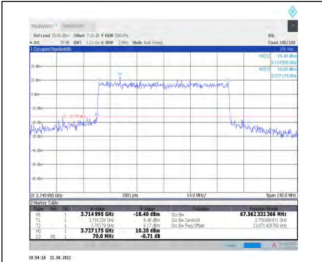
1-N78-3700-3800--30-70-M-7-CP-16QAM-Outer_Full -189@0-Ant1-67.562-70.000-≤70-PASS
