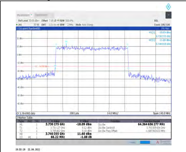
1-N78-3700-3800--30-70-H-3-DFT-16QAM-Outer_Fu II-180@0-Ant1-64.365-66.220-≤70-PASS
