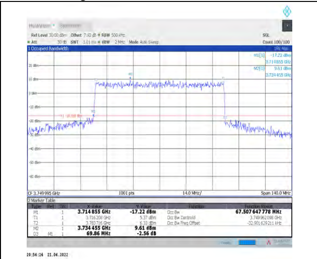
1-N78-3700-3800--30-70-M-8-CP-64QAM-Outer_Ful I-189@0-Ant1-67.508-69.860-≤70-PASS
