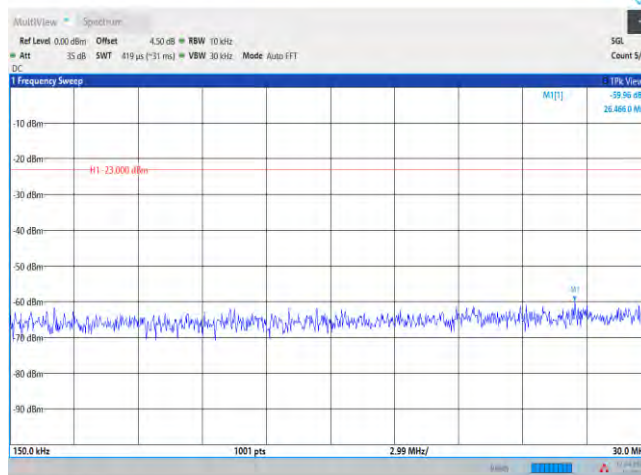
Band12-10MHz-QPSK-23060-1RB#0-Range2:0.15~30MHz
