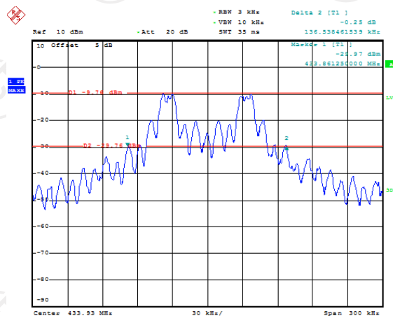
433.93MHz
