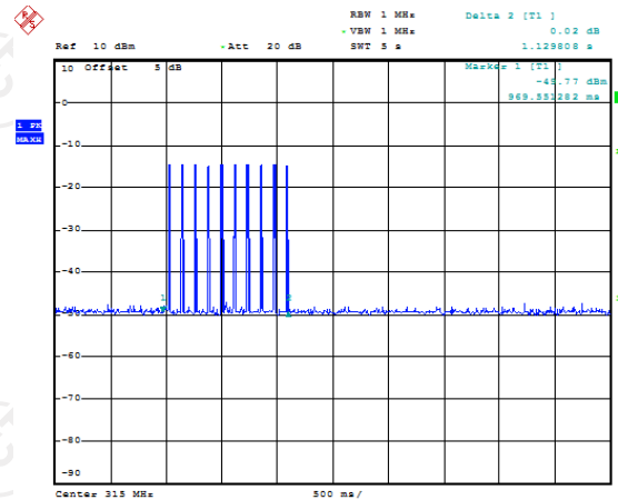
315MHz
