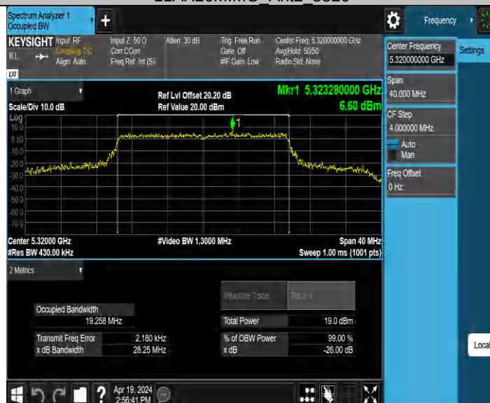
11AX20MIMO_Ant3_5320
