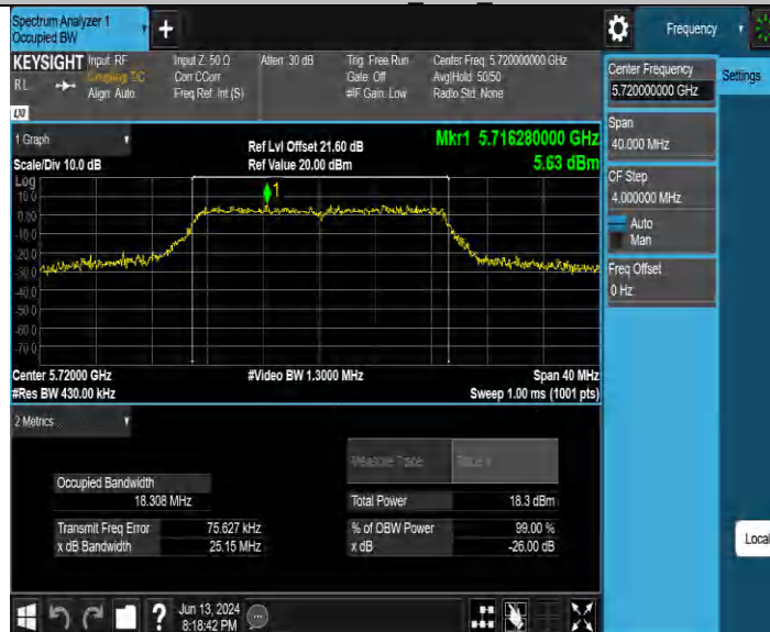
11AC20MIMO_Ant3_5720
