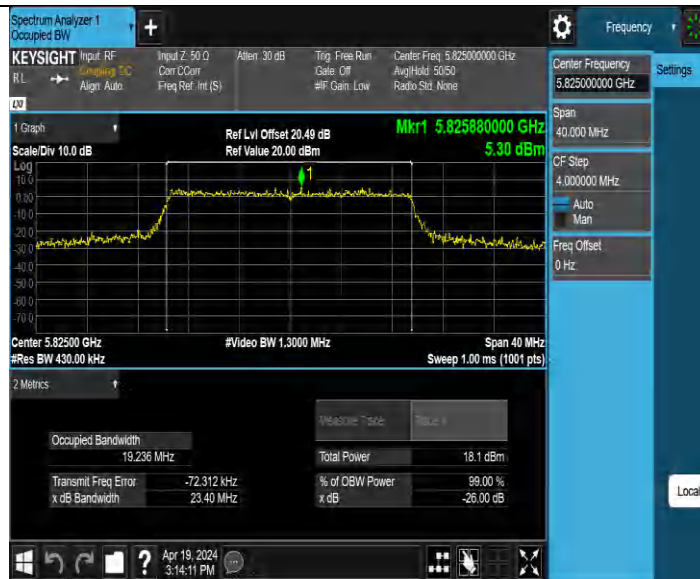
11AX20MIMO_Ant3_5825
