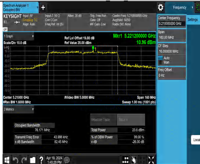
11AC80MIMO_Ant4_5210
