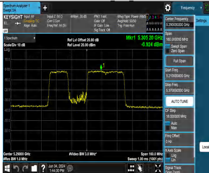
11BE80MIMO_Ant2 5290
