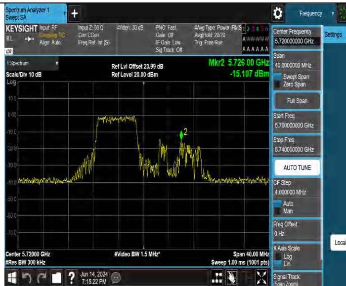
11BE20MIMO Ant3 5720 UNII-3 52+26 OFDMA 1
