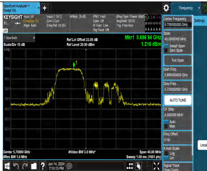
11BE20MIMO Ant2 5700 52+26 OFDMA 1
