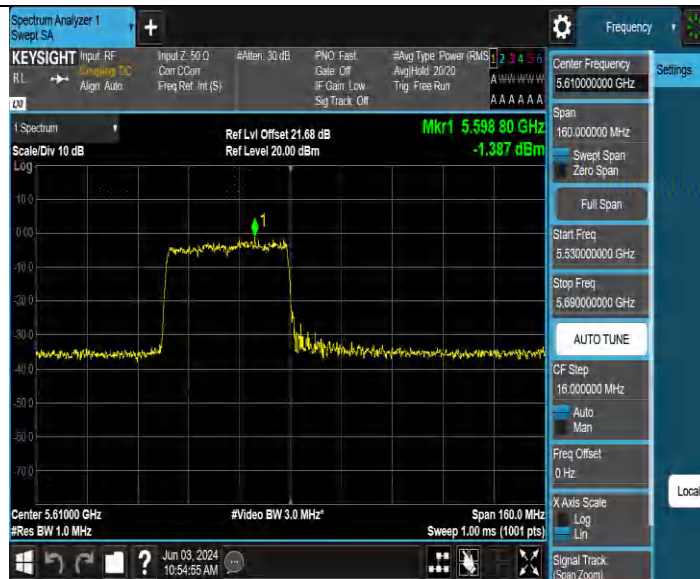
11BE80MIMO Ant4 5610 26Tone RU0
