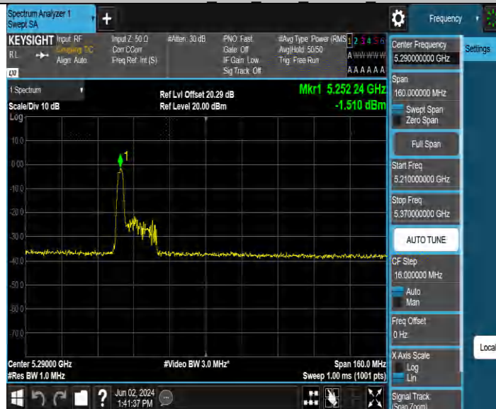
11BE80MIMO_Ant2_5290_484Tone_RU65
