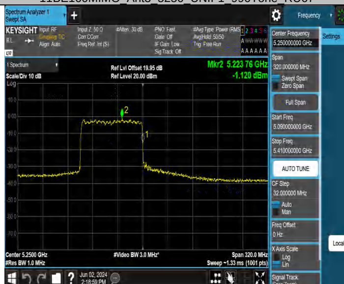
11BE160MIMO_Ant4 5250 UNII-1 996Tone RU67
