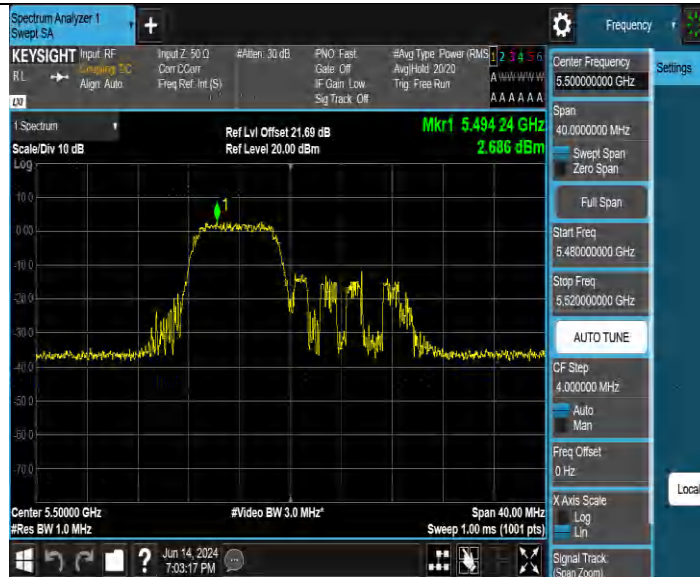
11BE20MIMO Ant4 5500 52+26 OFDMA 1
