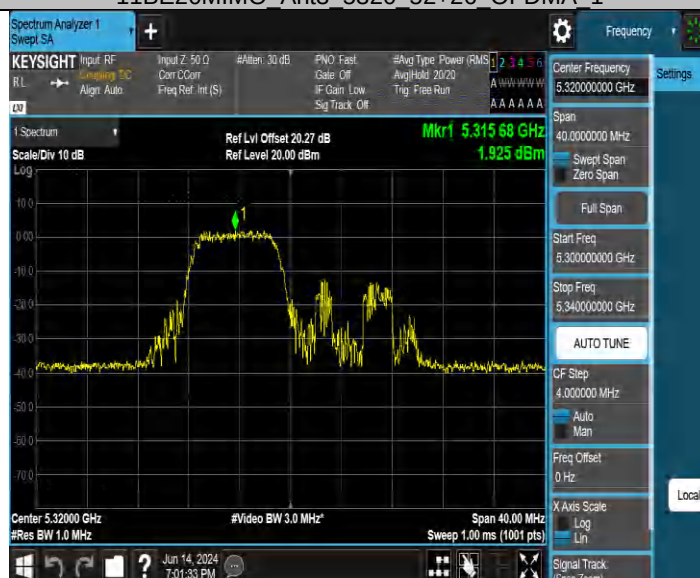
11BE20MIMO Ant4 5320 52+26 OFDMA 1
