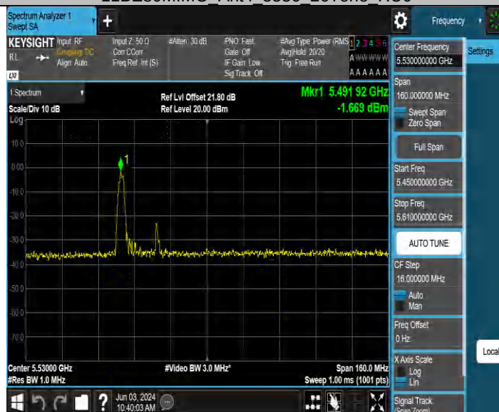
11BE80MIMO_Ant4 5530 484Tone RU65
