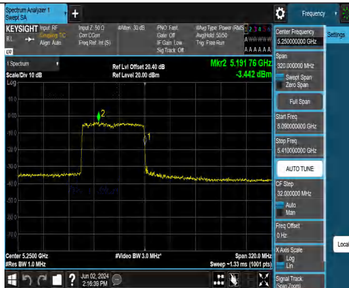
11BE160MIMO_Ant2 5250 UNII-1 996Tone RU67
