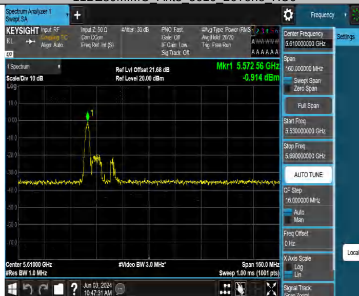
11BE80MIMO_Ant3_5610_484Tone_RU65
