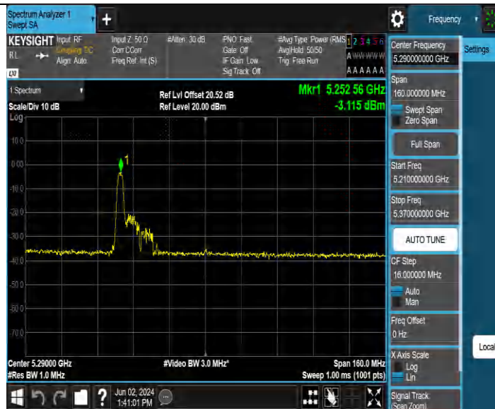
11BE80MIMO_Ant1_5290_484Tone_RU65
