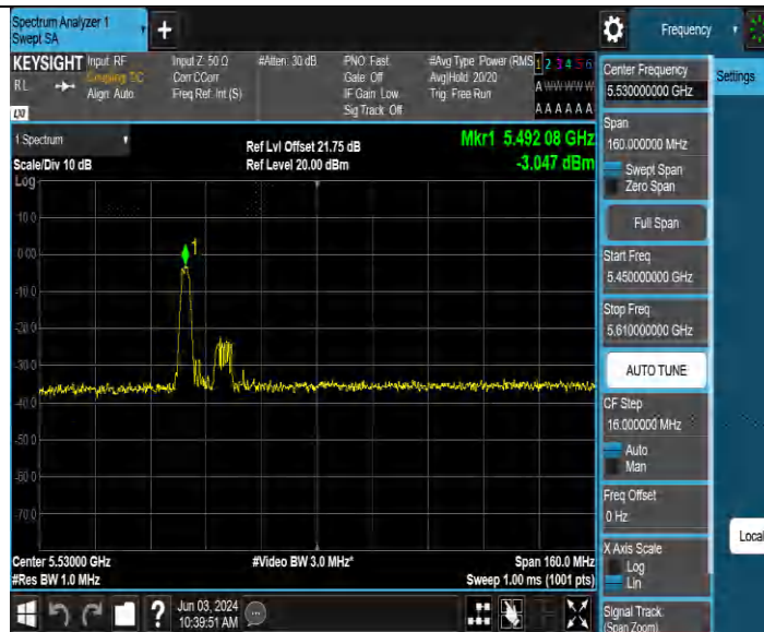
11BE80MIMO_Ant3 5530 484Tone RU65
