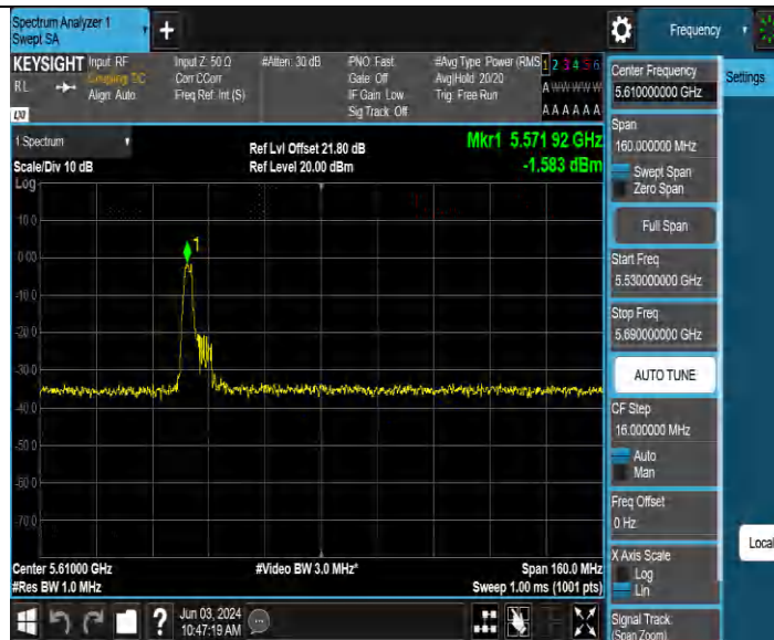
11BE80MIMO_Ant2_5610_484Tone_RU65
