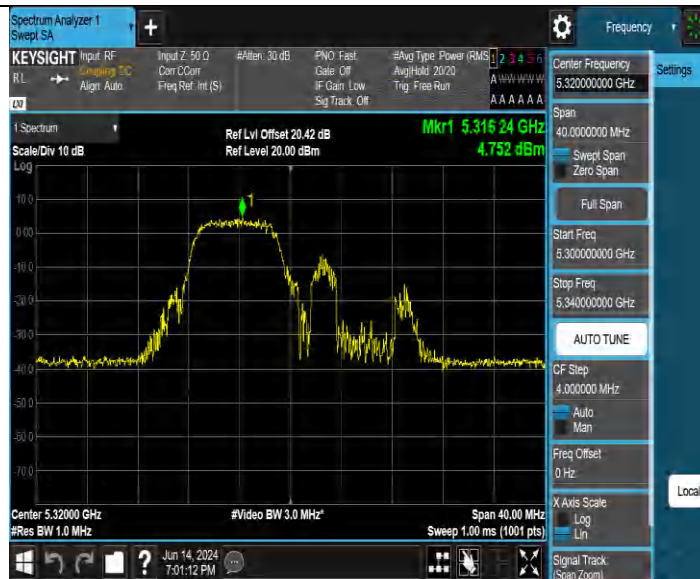
11BE20MIMO Ant2 5320 52+26 OFDMA 1
