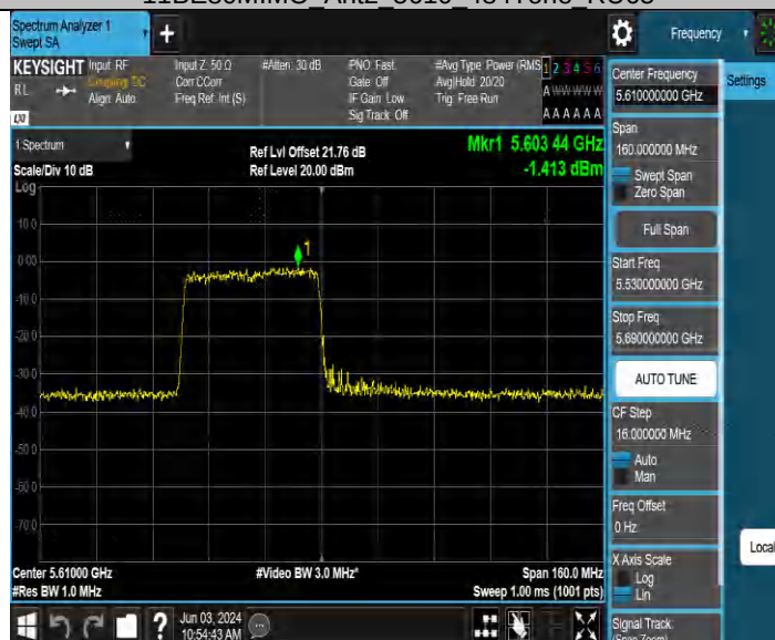
11BE80MIMO_Ant3_5610_26Tone_RU0
