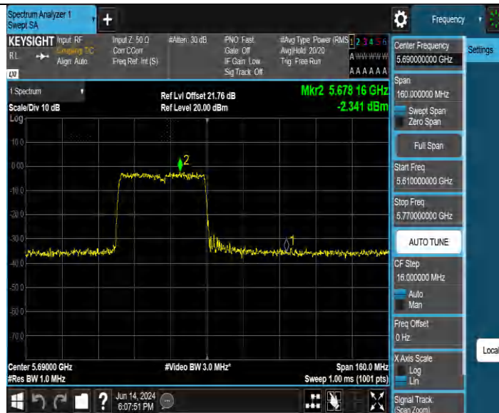
11BE80MIMO_Ant3_5690_UNII-2C_26Tone_RU0
