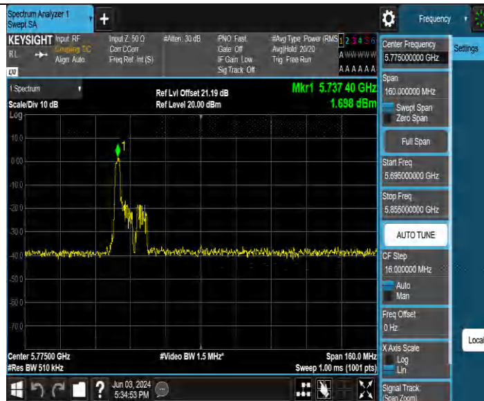
11BE80MIMO_Ant2_5775_484Tone_RU65
