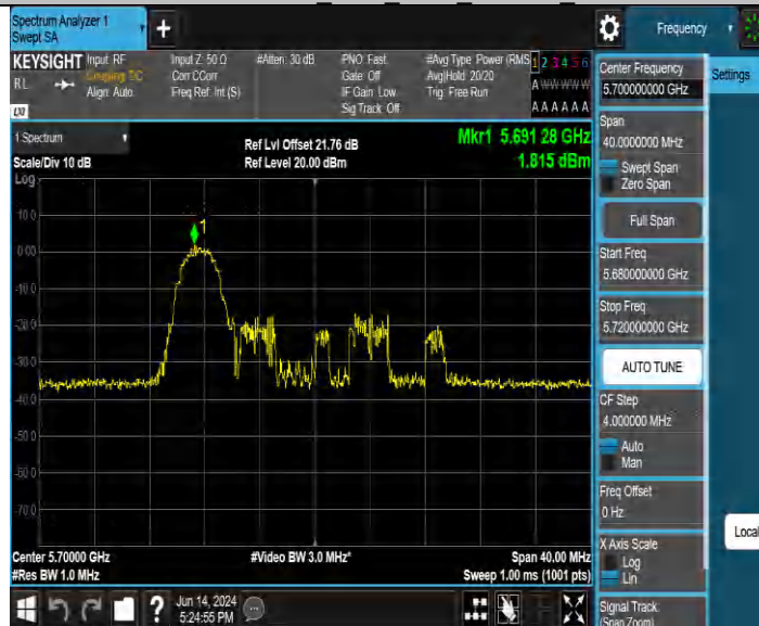
11BE20MIMO_Ant2_5700_106Tone_RU53
