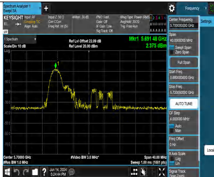
11BE20MIMO_Ant1_5700_106Tone_RU53
