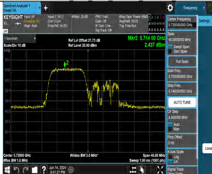
11BE20MIMO_Ant3_5720_UNII-2C_26Tone_RU0
