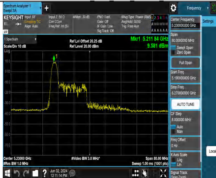
11BE40MIMO_Ant4_5230_242Tone_RU61
