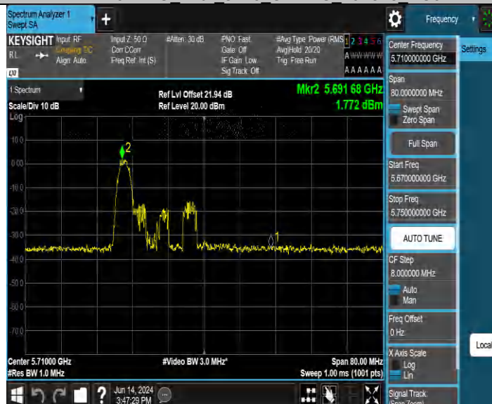
11AX40MIMO_Ant4_5710_UNII-2C_242Tone_RU61
