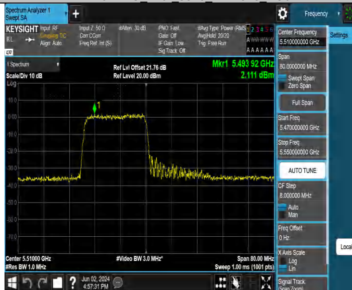
11AX40MIMO_Ant3_5510_26Tone_RU0
