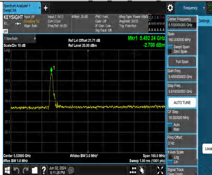
11AX80MIMO_Ant3_5530_484Tone_RU65
