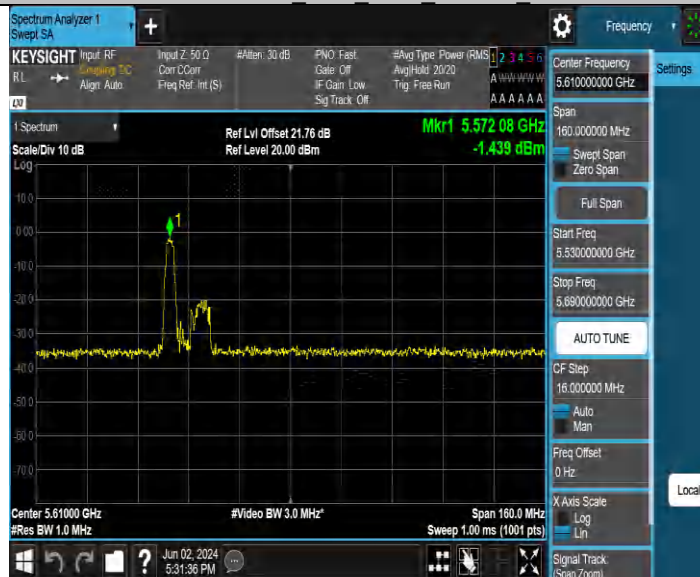
11AX80MIMO_Ant2 5610 484Tone RU65
