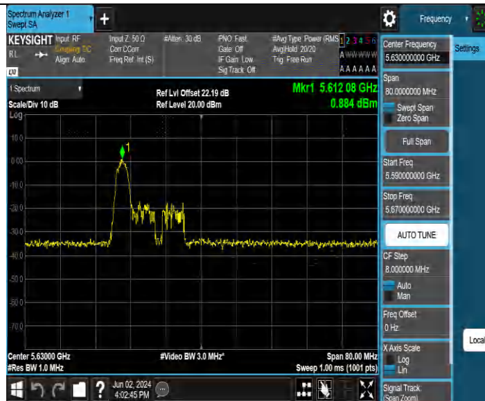
11AX40MIMO Ant1 5630 242Tone RU61
