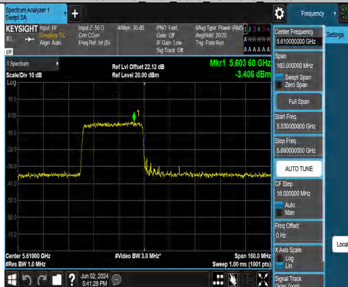
11AX80MIMO_Ant2 5610 26Tone RU0
