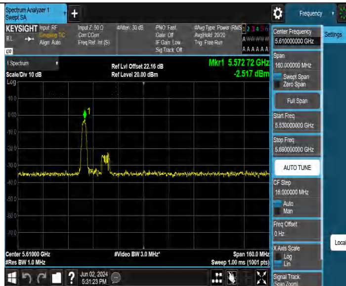
11AX80MIMO_Ant1 5610 484Tone RU65
