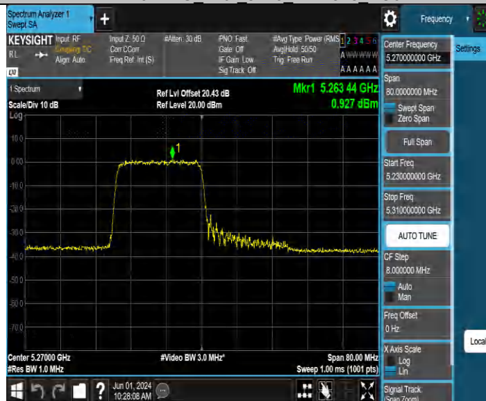
11AX40MIMO_Ant2_5270_26Tone_RU0
