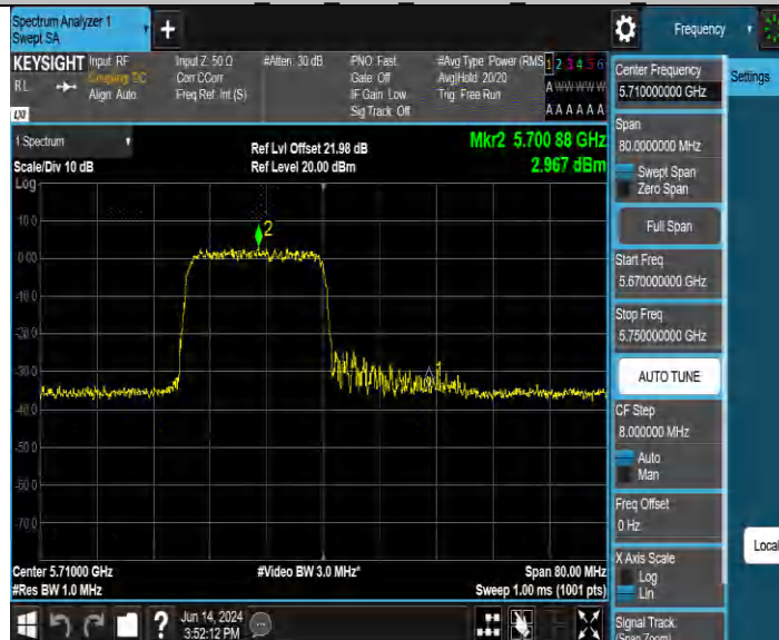
11AX40MIMO_Ant1_5710_UNII-3_26Tone_RU0
