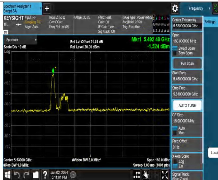
11AX80MIMO_Ant2_5530_484Tone_RU65
