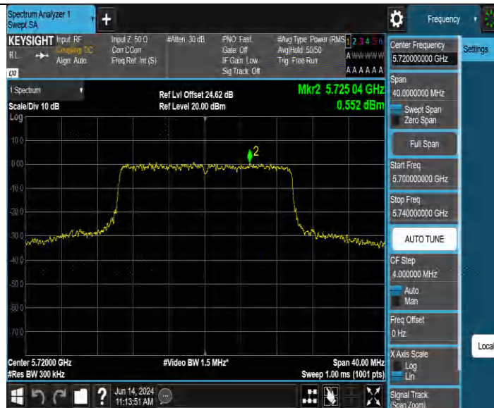
11BE20MIMO Ant2 5720 UNII-3
