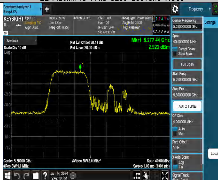
11AX20MIMO Ant4 5280 26Tone RU0
