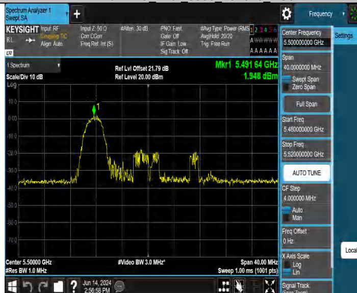
11AX20MIMO Ant4 5500 106Tone RU53
