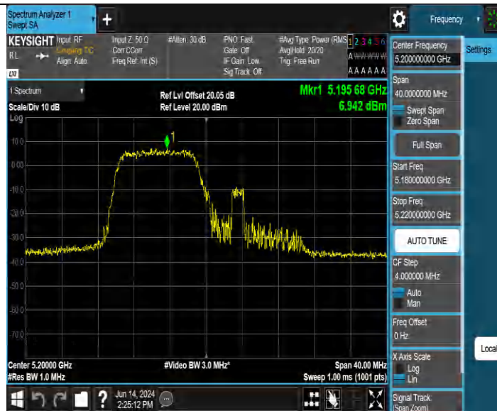
11AX20MIMO Ant3 5200 26Tone RU0
