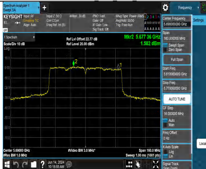
11AC80MIMO_Ant4_5690_UNII-2C
