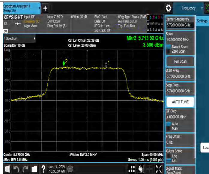
11AX20MIMO_Ant2_5720_UNII-2C
