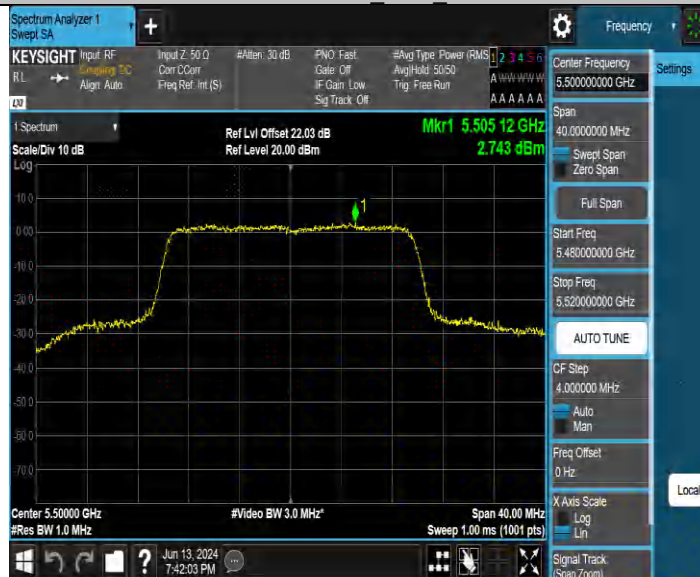
11AX20MIMO_Ant4_5500
