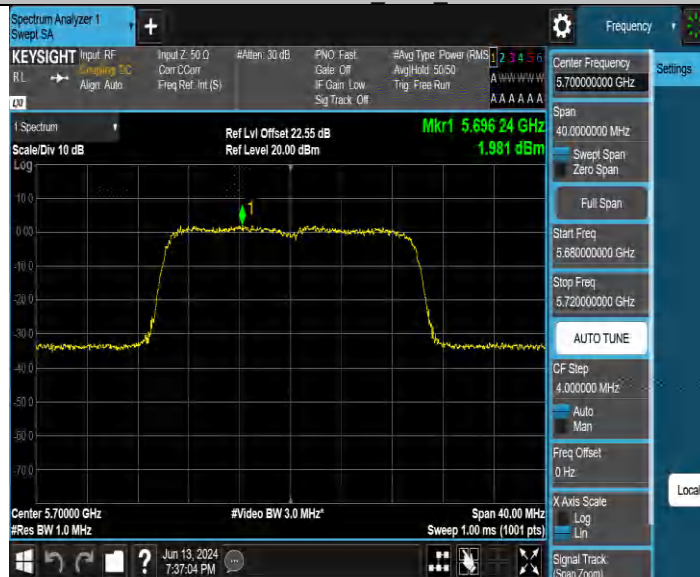
11AC20MIMO_Ant4 5700
