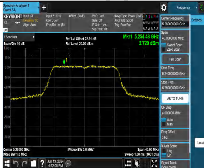
11N20MIMO Ant4 5260
