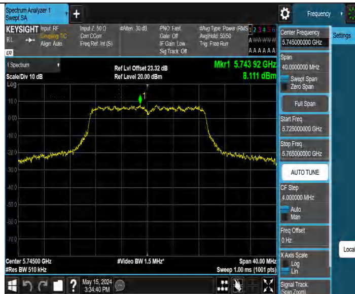
11N20MIMO Ant3 5745
