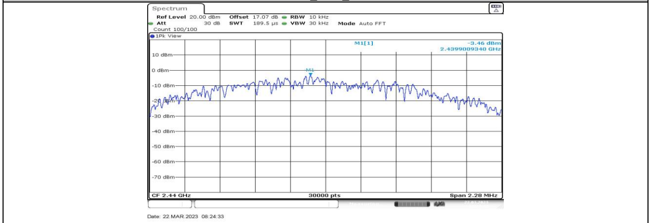
LE 2M_Ant1_2440
