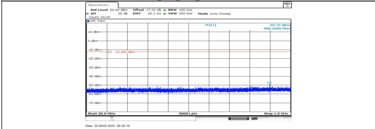
LE 2M_Ant1_2480_30~1000
