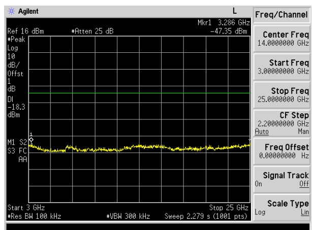
3GHz-25GHz
