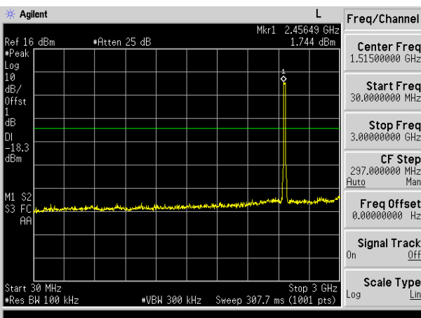
30MHz-3GHz
