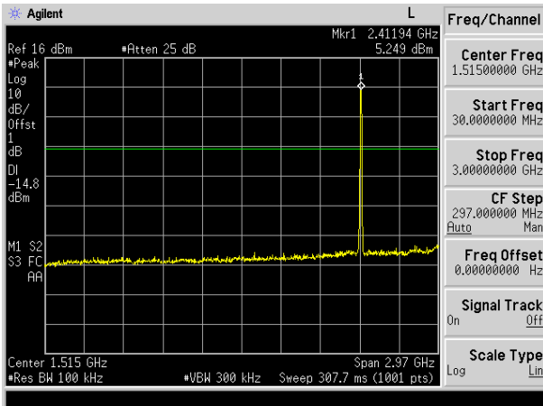
30MHz-3GHz
