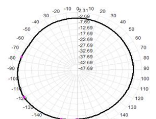
2470.0MHz Total(H), Max= 0.74dBi
