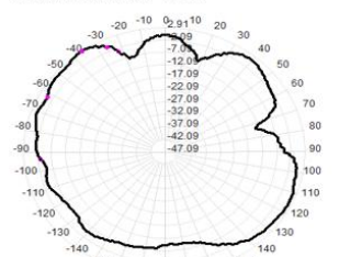
2470.0MHz Total(E1), Max= 3.39dBi
