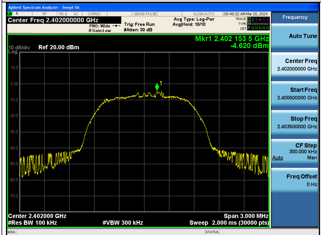
Test_Graph_EDR_ANT1_2402_2Mbps_Reference Level
