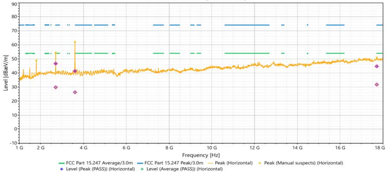
#2 - 1GHz-18GHz (Horizontal)
