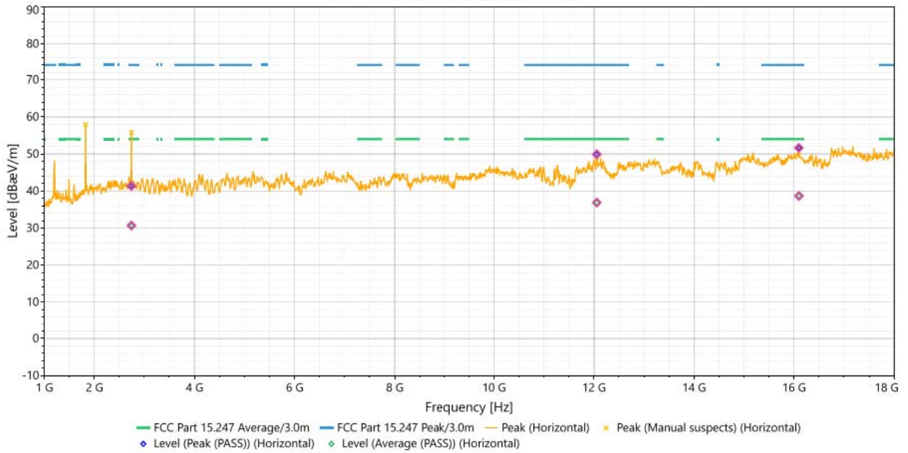
#2 - 1GHz-18GHz (Horizontal)
