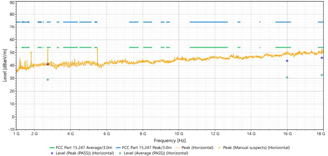
#2 - 1GHz-18GHz (Horizontal)
