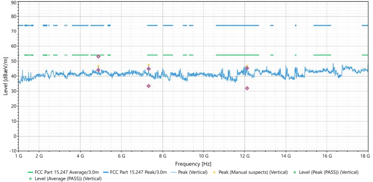
#1 - 1GHz-18GHz (Vertical)
