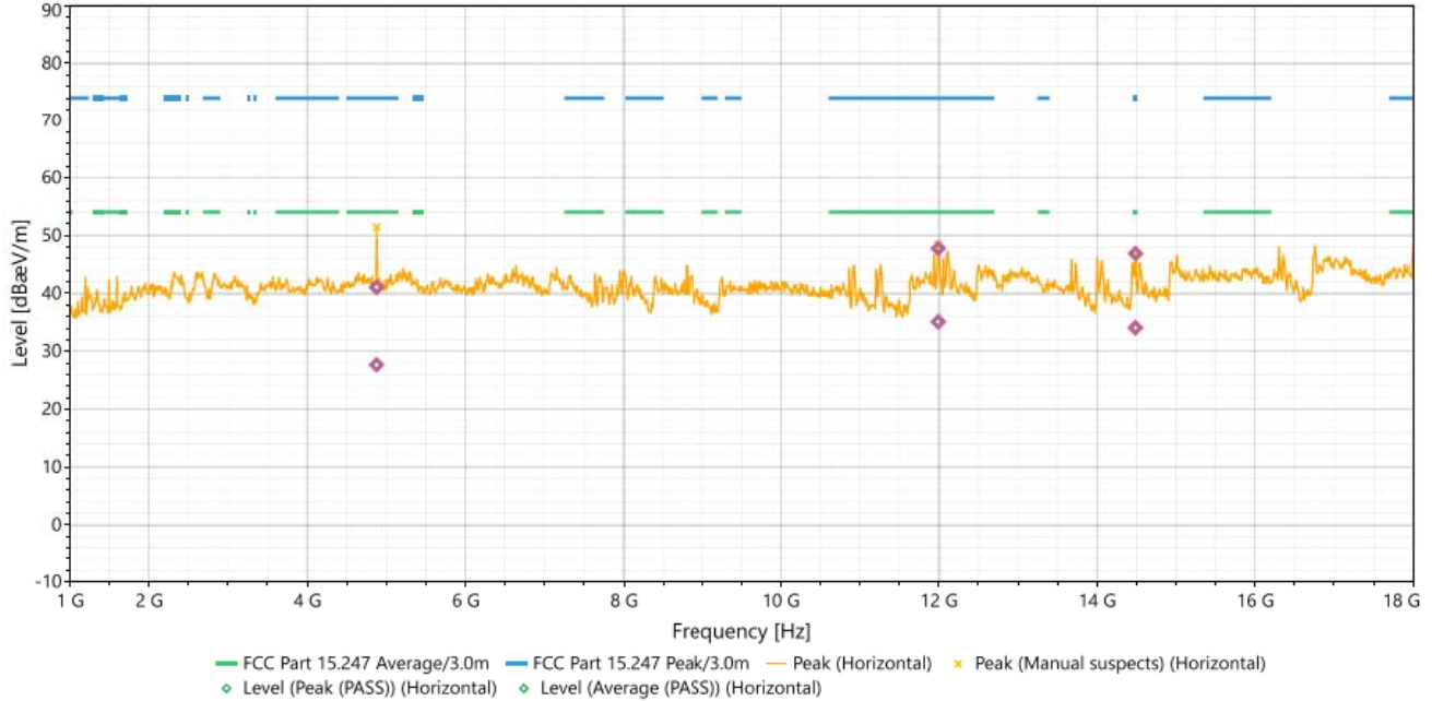
#2 - 1GHz-18GHz (Horizontal)
