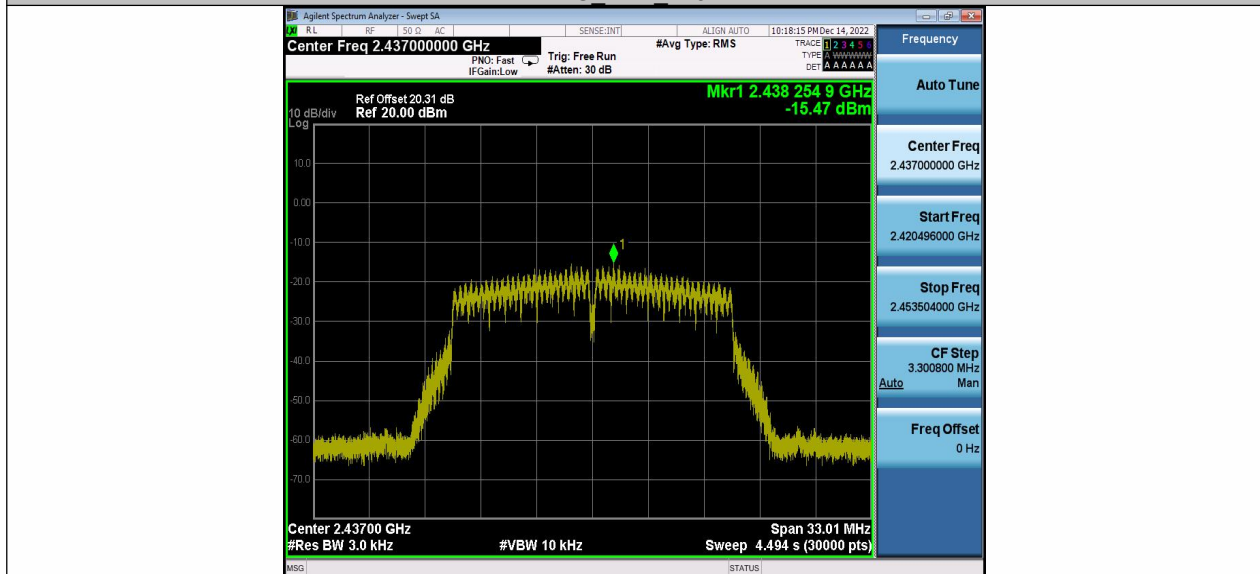
11G_Ant2_2437
