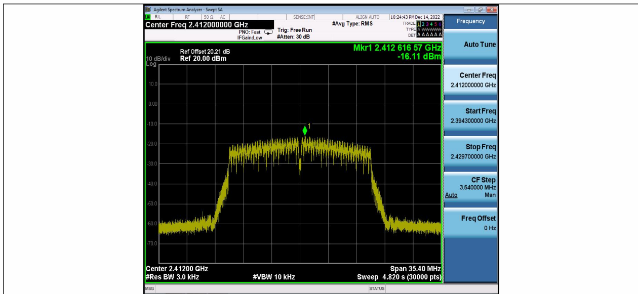
11N20MIMO_Ant2_2412
