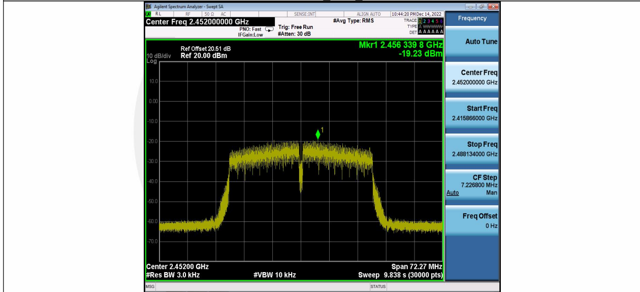
11N40MIMO_Ant2_2452
