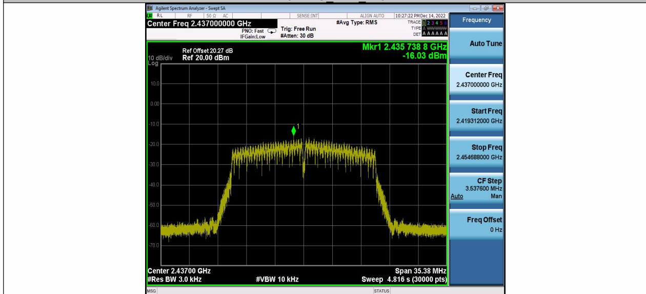
11N20MIMO_Ant1_2437
