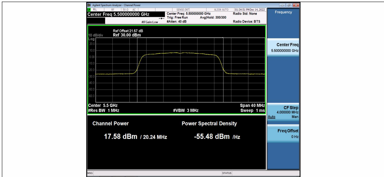
11N20MIMO_Ant2_5500
