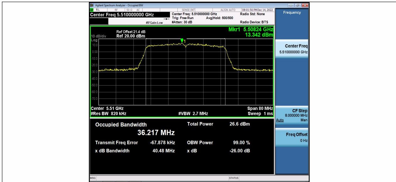
11AC40MIMO_Ant2_5510
