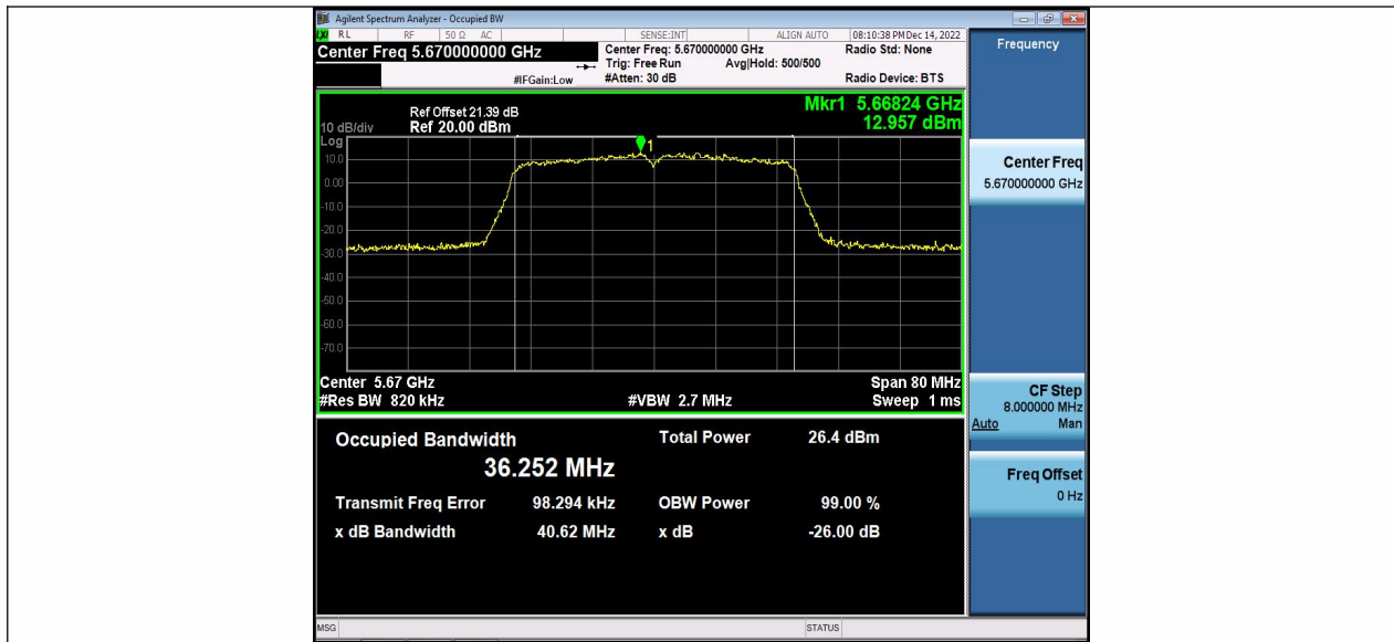
11AC40MIMO_Ant2_5670
