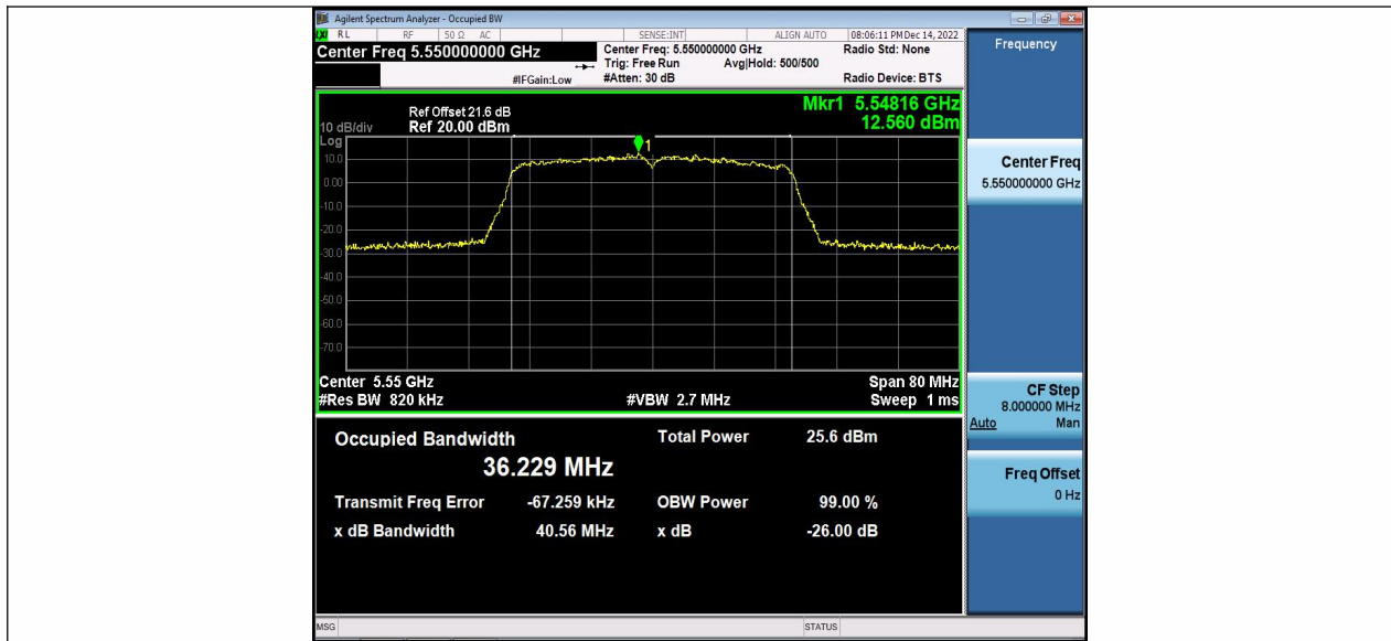
11AC40MIMO_Ant2_5550
