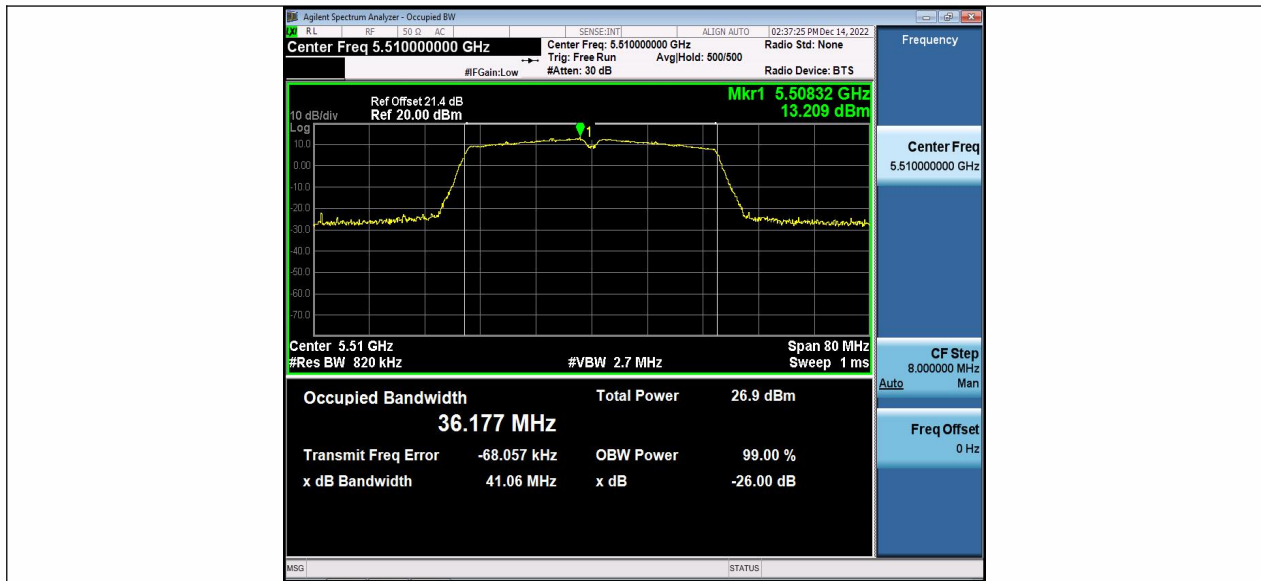
11N40MIMO_Ant2_5510
