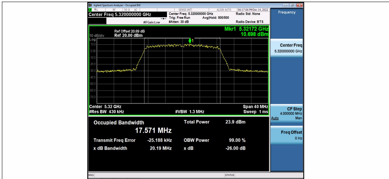
11AC20MIMO_Ant2_5320
