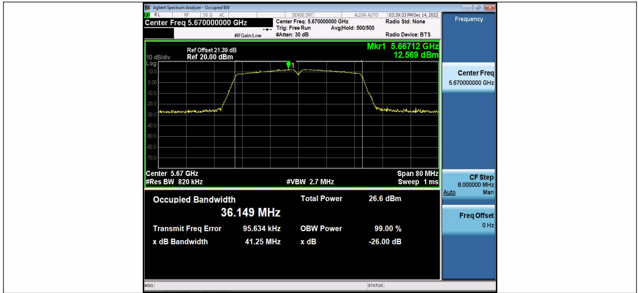
11N40MIMO_Ant2_5670
