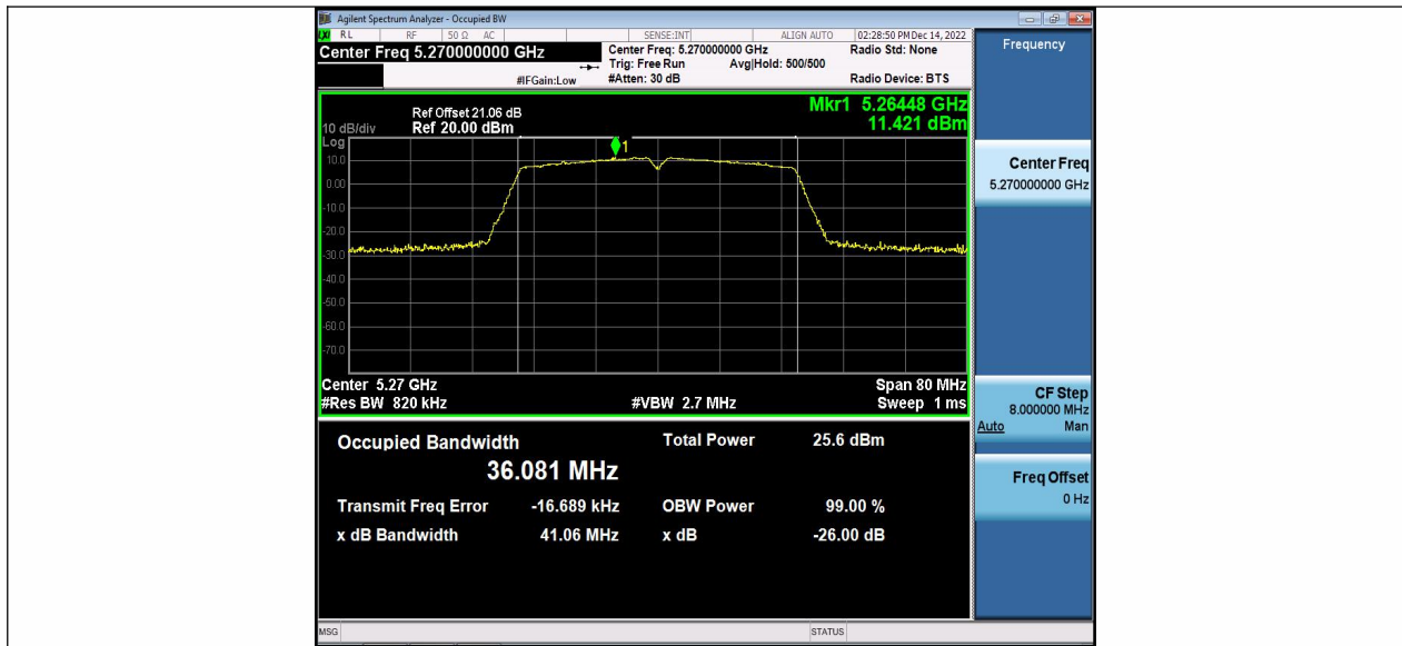
11N40MIMO_Ant2_5270
