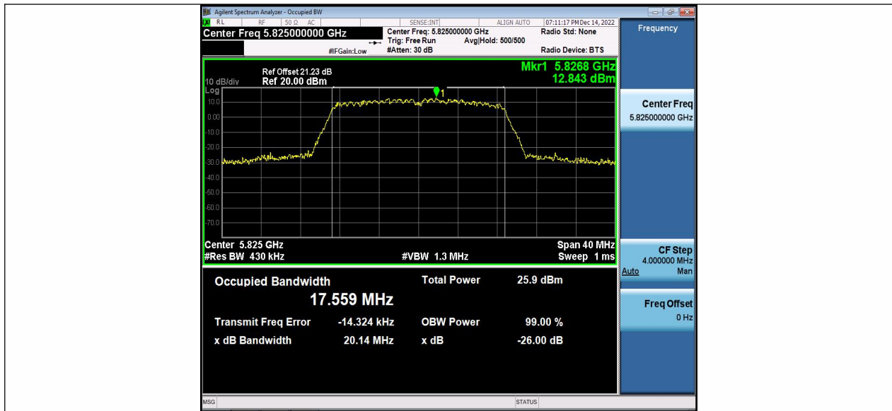
11AC20MIMO_Ant2_5825
