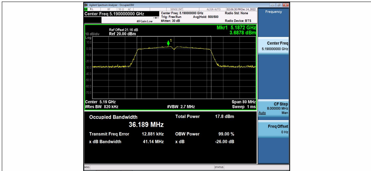
11N40MIMO_Ant2_5190
