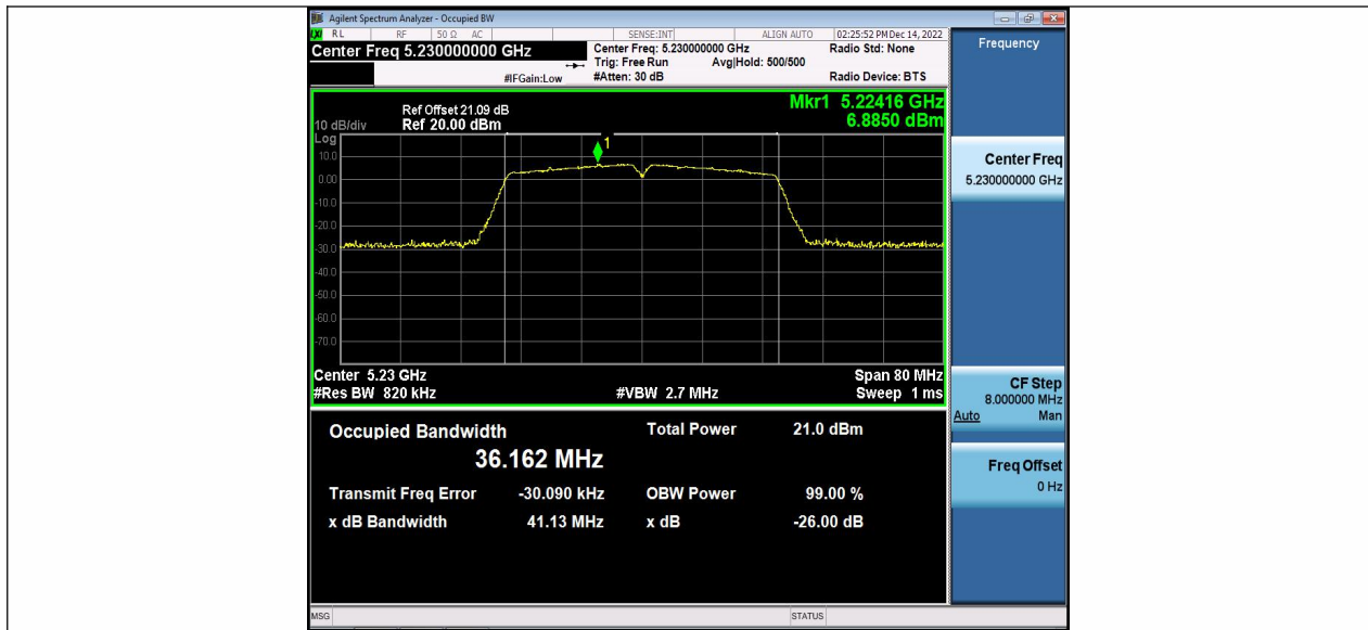
11N40MIMO_Ant2_5230
