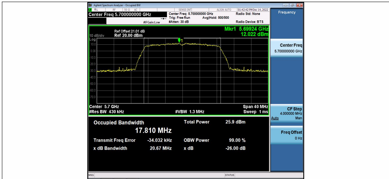
11N20MIMO_Ant2_5700
