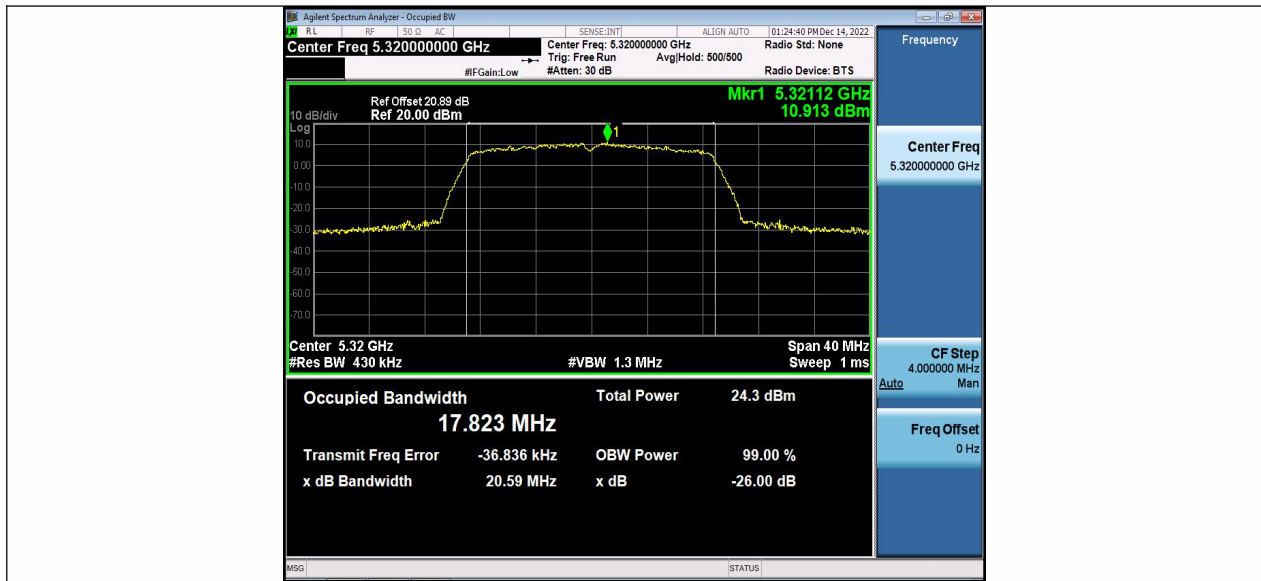
11N20MIMO_Ant2_5320
