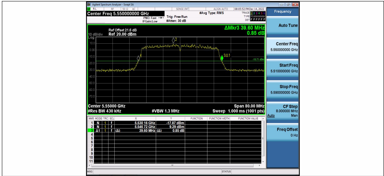
11AC40MIMO_Ant2_5550
