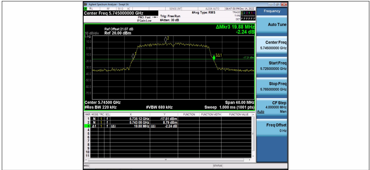
11AC20MIMO_Ant2_5745
