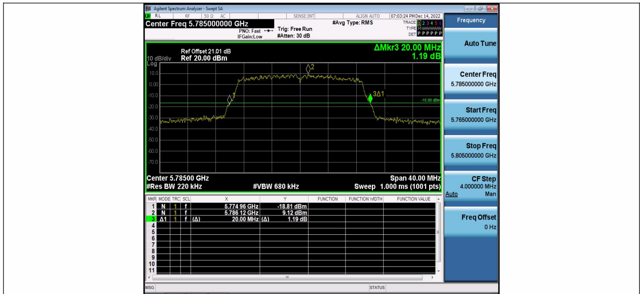
11AC20MIMO_Ant2_5785
