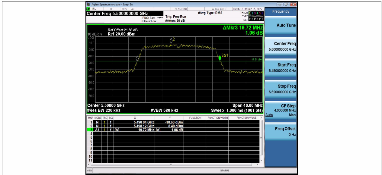
11AC20MIMO_Ant2_5500
