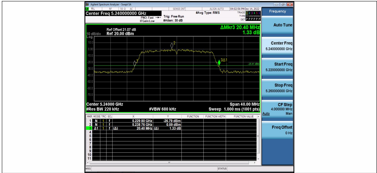
11AC20MIMO_Ant2_5240
