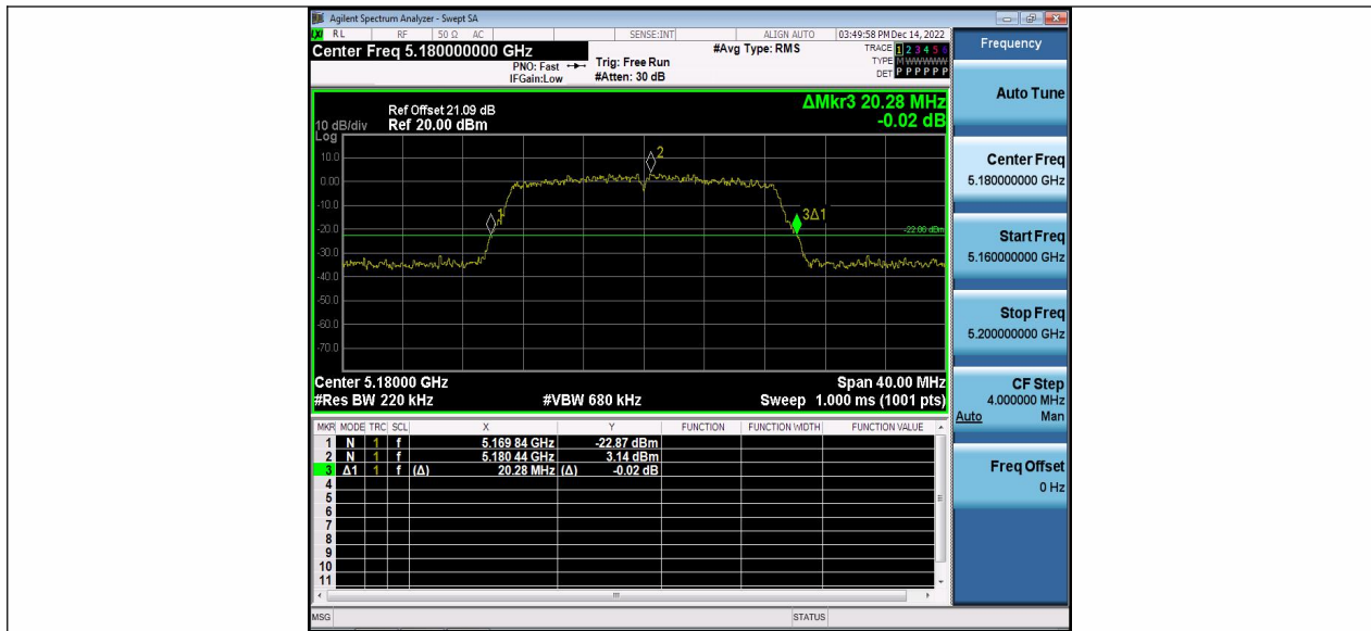
11AC20MIMO_Ant2_5180
