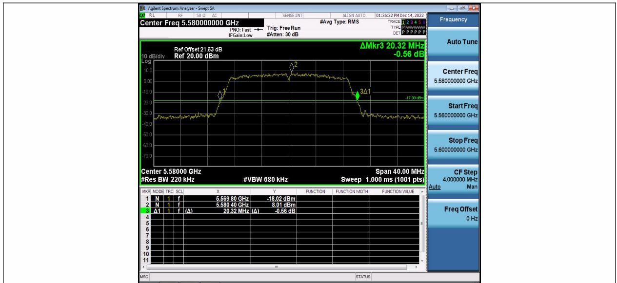
11N20MIMO_Ant2_5580
