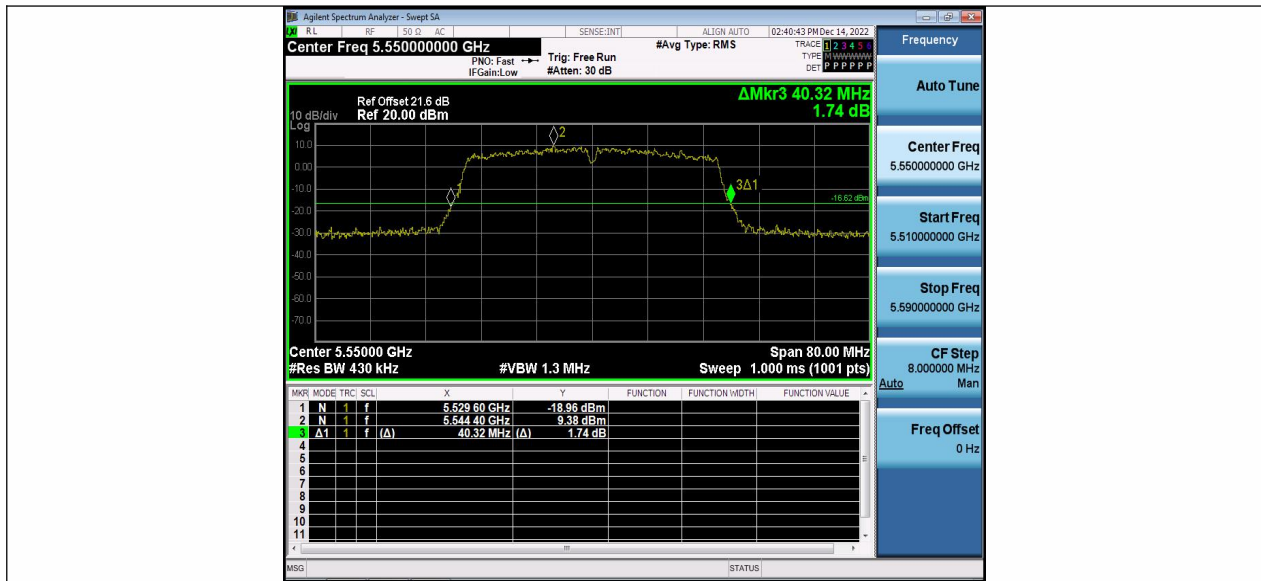
11N40MIMO_Ant2_5550
