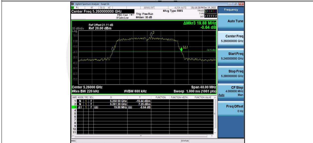
11N20MIMO_Ant1_5280
