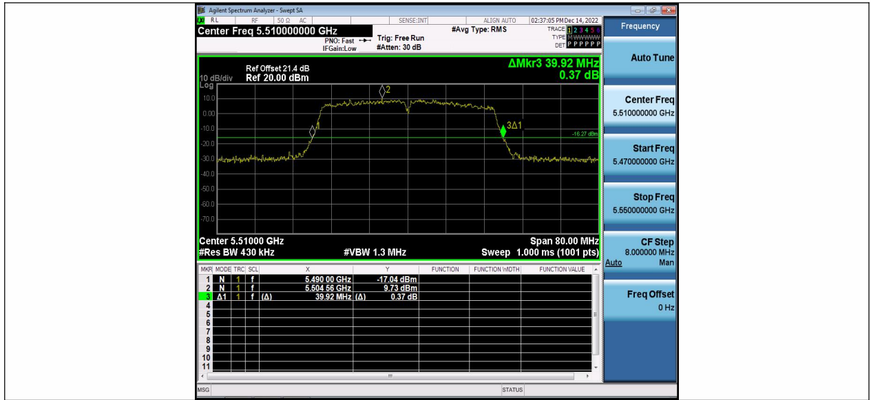
11N40MIMO_Ant2_5510
