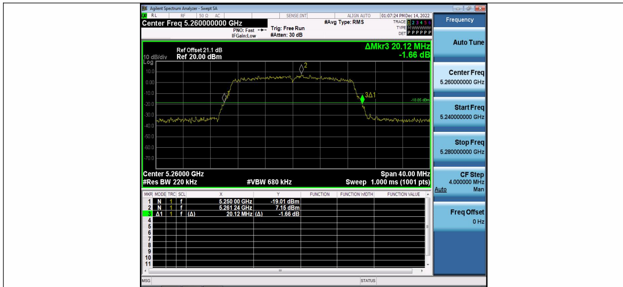
11N20MIMO_Ant2_5260
