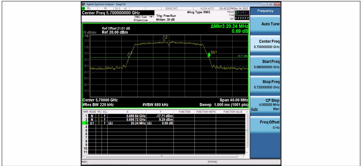
11N20MIMO_Ant2_5700
