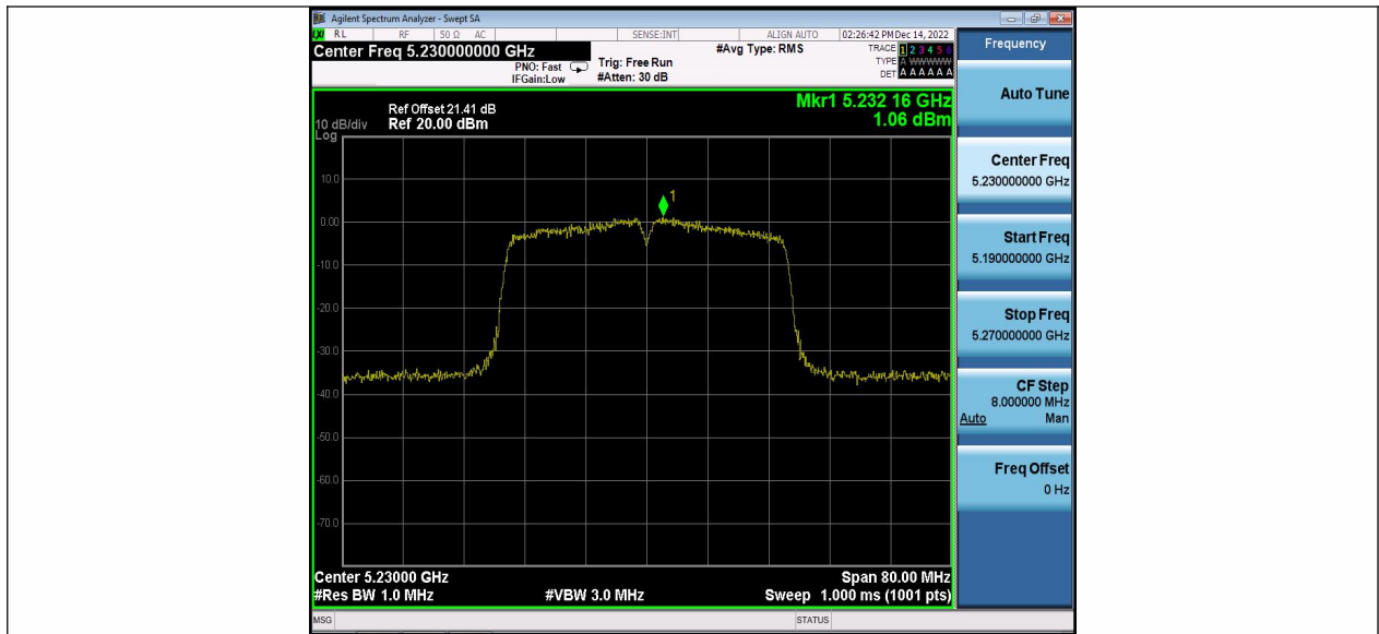
11N40MIMO_Ant2_5230
