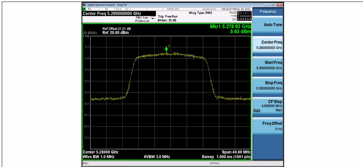
11N20MIMO_Ant2_5280
