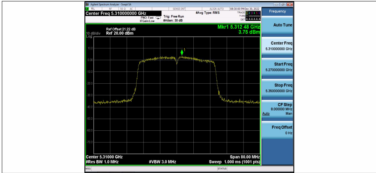
11N40MIMO_Ant2_5310
