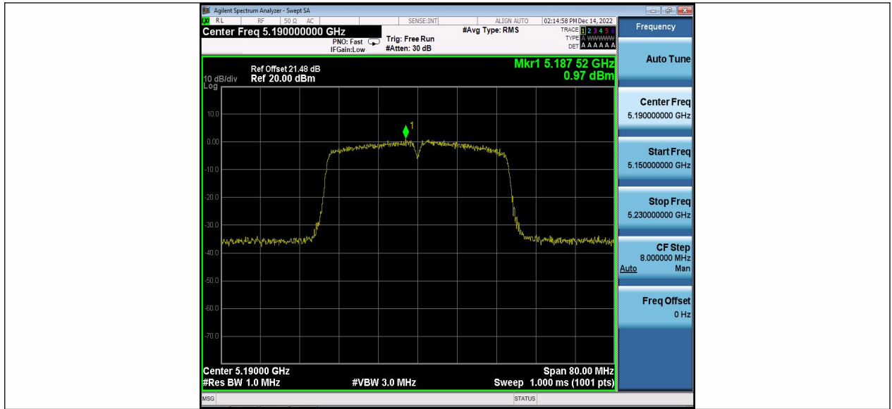
11N40MIMO_Ant2_5190
