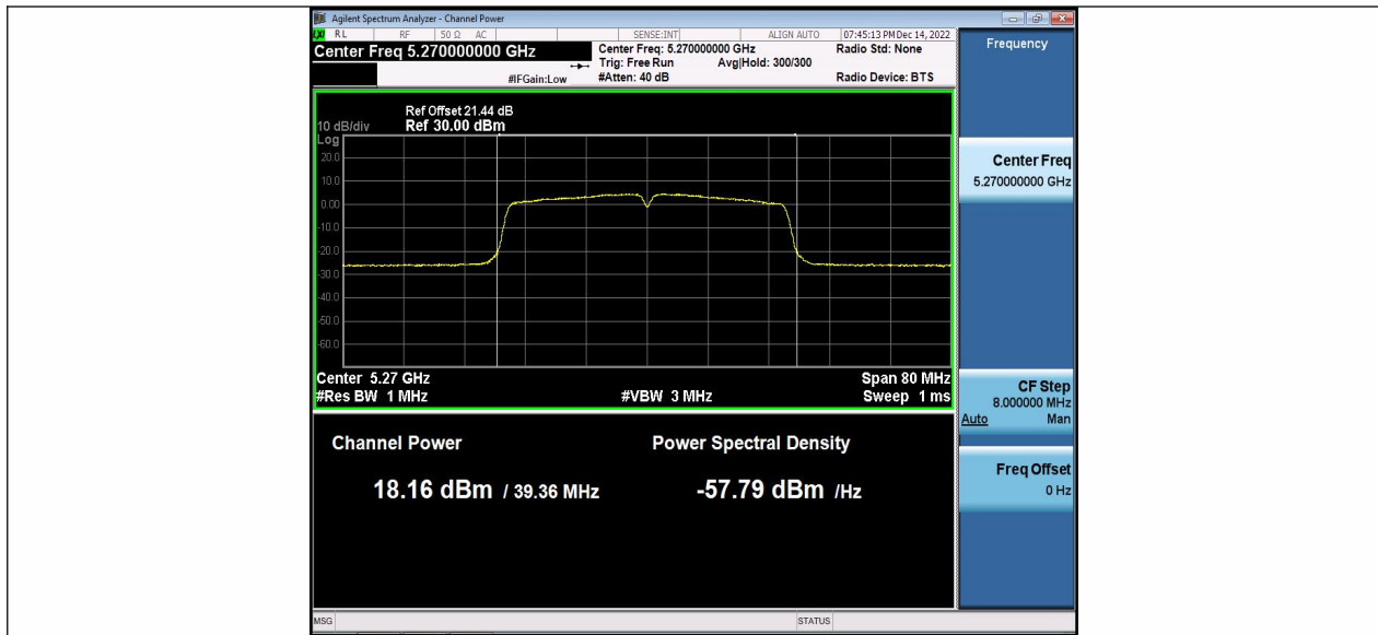
11AC40MIMO_Ant2_5270
