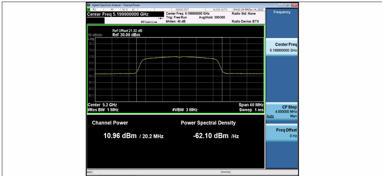
11AC20MIMO_Ant2_5200
