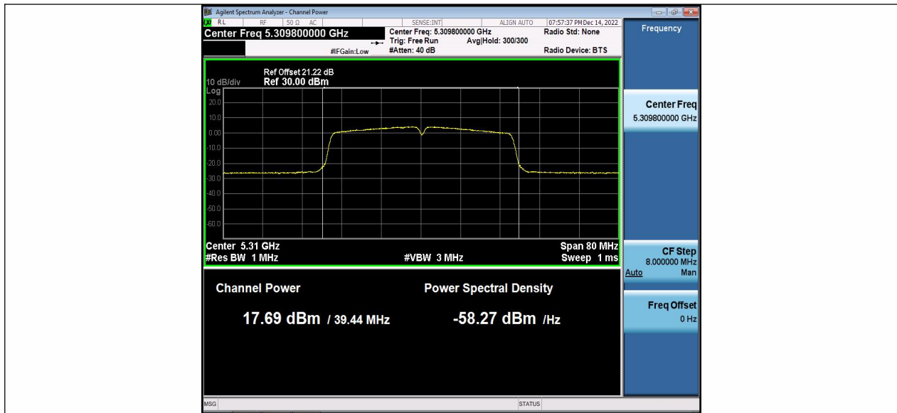
11AC40MIMO_Ant2_5310
