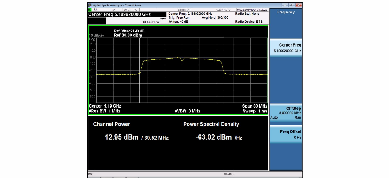
11AC40MIMO_Ant2_5190
