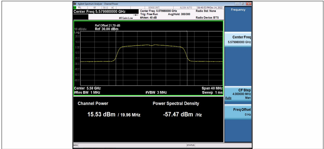
11AC20MIMO_Ant2_5580
