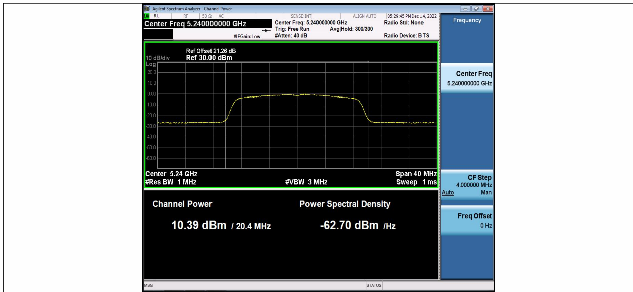
11AC20MIMO_Ant2_5240
